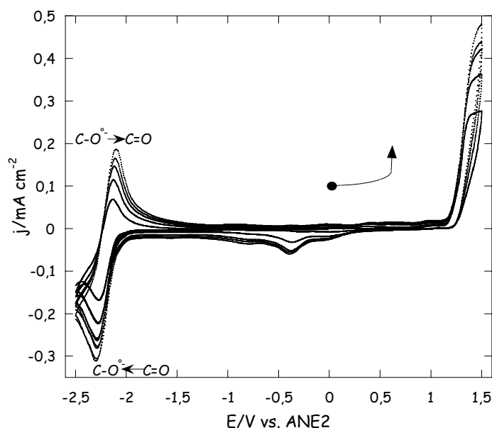
Figure B 6 : Voltampérométrie à 80°C après barbotage d'argon de l'EC à 0,1 mol·L -1 à différentes vitesses de balayage v_b = 100, 200, 300, 400 et 500 \text{ mV}\cdot\text{s}^{-1} pour les courbes suivant respectivement les courants croissants (en valeur absolue).
