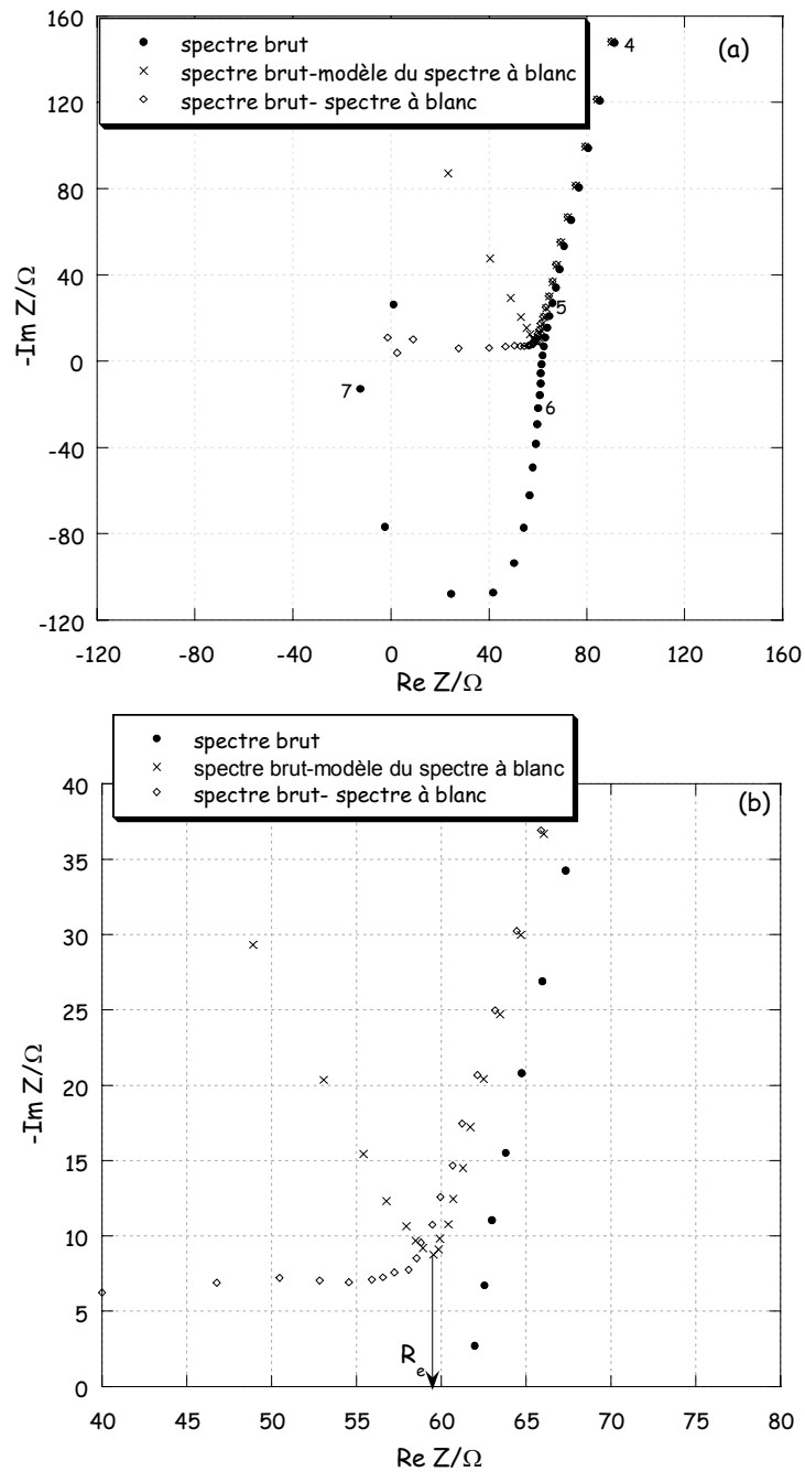
Figures E 8 : Spectre d'impédance brut du Nafion ® 117 au point (20°C, 100%HR dans l'eau), en soustrayant le modèle du spectre à blanc ou le spectre à blanc, aux hautes fréquences (a) et réduit aux fréquences intéressants la détermination de la résistance de l'électrolyte (b), paramétré en logarithme décimal de la fréquence.
