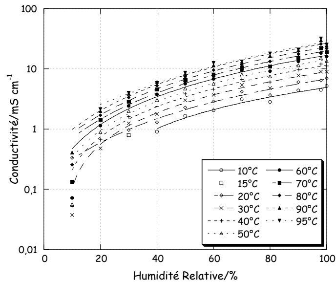
Figure E 14 : Isothermes de conductivités du Nafion ® 117 en fonction de l'humidité relative.
