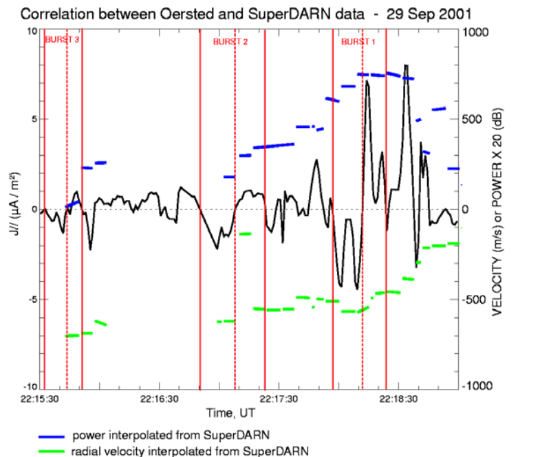
Fig. 7.11 : Événement du 29 septembre 2001. Courant aligné mesuré par Ørsted, en fonction du temps. La vitesse radiale (segments verts) et la puissance du signal rétrodiffusé (segments bleus) mesurées par le radar de Kodiak au niveau de la projection d'Ørsted et interpolées sur les trois cartes encadrant le passage, sont également tracées. Les courants associés aux trois sursauts sont délimités par les lignes rouges
