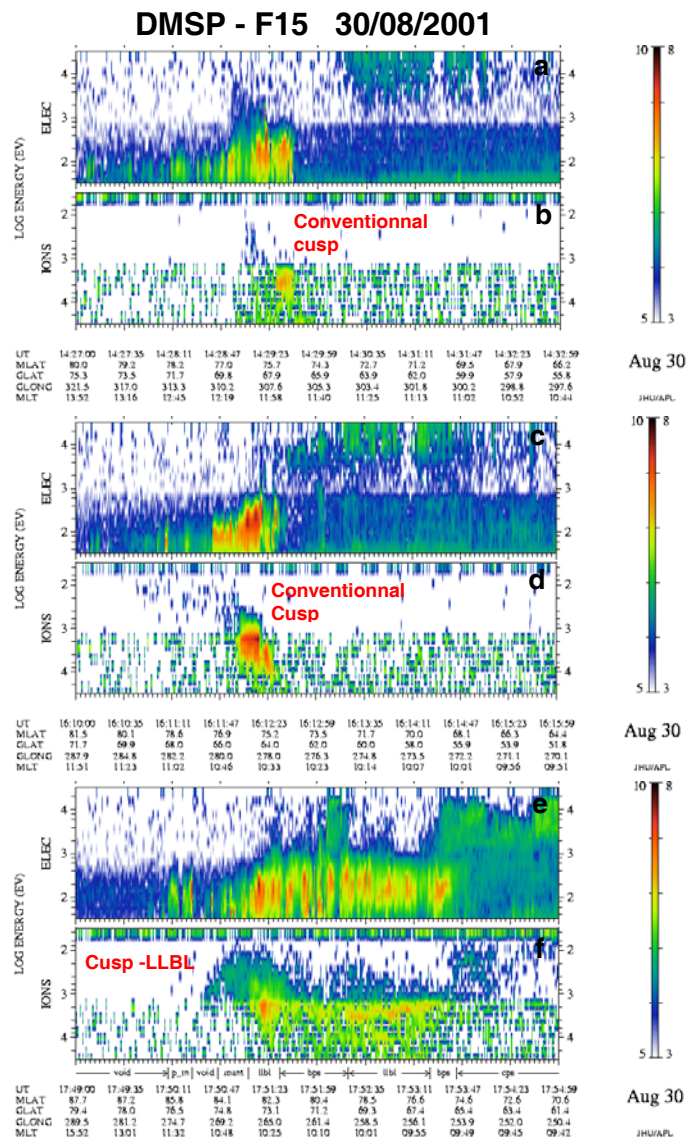
Fig. 5.6 : Evénement du 30/08/2001. Spectrogrammes des flux des électrons et des ions en fonction du temps et de l'énergie, pour les trois passages de DMSP F-15. A noter, que les ions de basse énergie ne sont pas mesurés par le satellite DMSP-F15.
