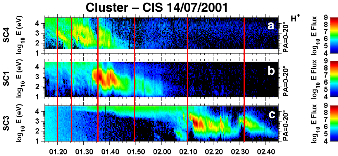
Fig. 6.5 : Evénement du 14/07/2001. Spectrogrammes (temps, énergie) des flux des ions H^+ , mesurés par Cluster-CIS dans la direction parallèle au champ magnétique (angle d'attaque = 0-20^\circ ), pour les satellites 4-1-3, sur la période 01:15-02:45 TU. Les lignes rouges verticales correspondent aux temps initiaux des différentes dispersions d'ions.
