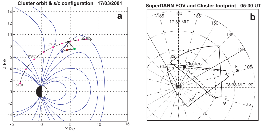
Fig. 4.1 : Evénement du 17/03/2001 (a) Schéma de la projection de l'orbite de Cluster-1 (ligne noire) dans le plan XZ GSM, sur la période 01:00-09:00 TU, le 17 mars 2001. Les points roses le long de l'orbite sont séparés par 1h TU. La configuration du tétraèdre Cluster est représentée vers 06:45 TU, chaque satellite étant représenté par un point coloré (C1-noir, C2-rouge, C3-vert, C4-bleu). La séparation entre les satellites a été agrandie d'un facteur 10. Quelques lignes magnétosphériques (lignes bleues) ont également été tracées. (b) Champs de vue communs en coordonnées magnétiques des radars SuperDARN d'Hankasalmi (F) et de Thikkvibaer (E), représentés à 05:30 TU. Le faisceau 14 d'Hankasalmi et le faisceau 2 de Thikkvibaer sont superposés aux champs de vue (lignes pointillées), ainsi que la projection de Cluster (point noir).
