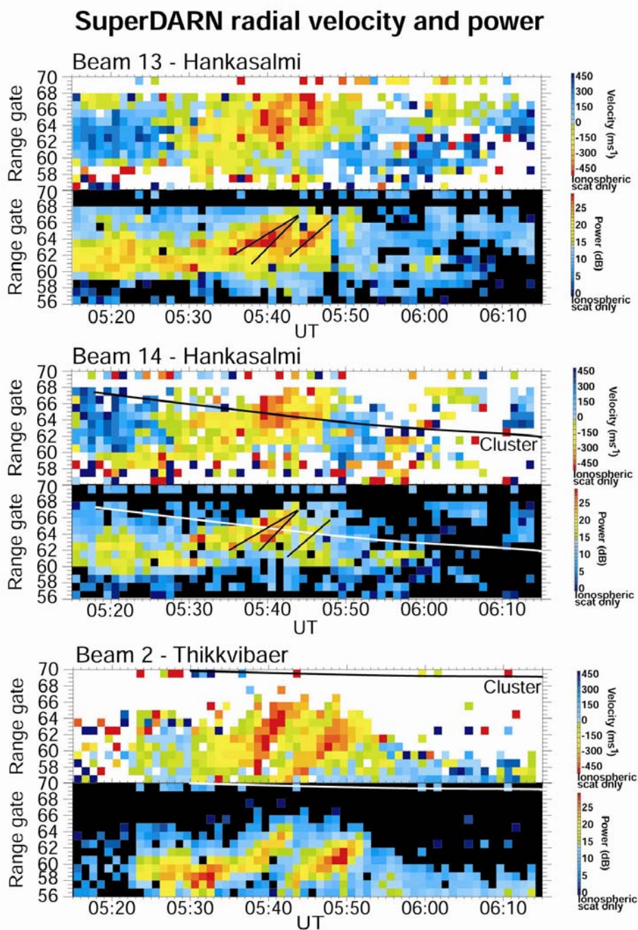
Fig. 4.4 : Événement du 17/03/2001. Paires de diagrammes temps-distance pour la vitesse radiale et pour la puissance rétrodiffusée du signal, pour trois faisceaux SuperDARN, sur la période 05:15-06:15 TU. La projection de Cluster est superposée au faisceau 14 d'Hankasalmi et au faisceau 2 de Thikkvibaer (lignes noires ou blanches). La pente des structures de forte puissance, dispersées au cours du temps est représentée sous forme de segments noirs sur les diagrammes de puissance des faisceaux 13 et 14 d'Hankasalmi.
