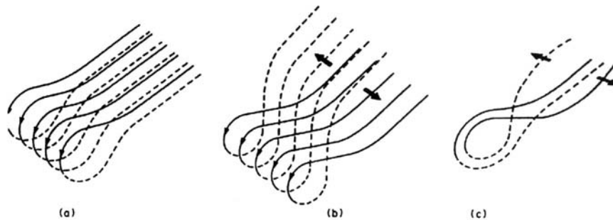
Fig. 2.3 : (a) Lignes de champ magnétique récemment reconnectées à la magnétopause (avec les lignes pointillées du côté de la magnétosphère). (b) La présence d'un cisaillement de vitesse déforme les lignes de champ à travers la magnétopause. (c) Deux lignes de champ reconnectées, la plus interne a été reconnectée la première et est donc plus déformée (d'après Southwood et al. , 1988).
