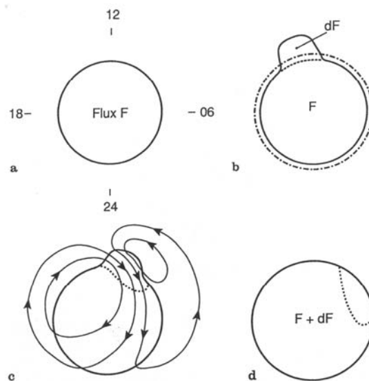
Fig. 2.6 : Mêmes schémas que sur la figure 2.5 illustrant la réponse de la convection à une impulsion de la reconnexion magnétique, en présence d'une composante matin-soir positive de l'IMF, dans l'hémisphère nord (d'après Cowley et Lockwood, 1992).
