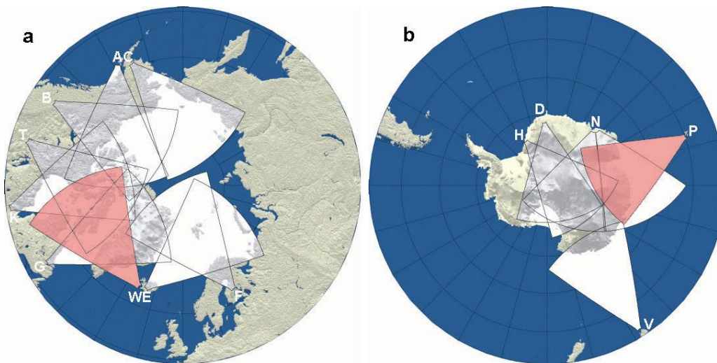
Fig. 3.1 : Les champs de vue des radars SuperDARN. (a) dans l'hémisphère nord. (b) dans l'hémisphère sud. Les champs de vue des radars français en Islande (W) et aux Iles Kerguelen (P) sont représentés en rouge.
