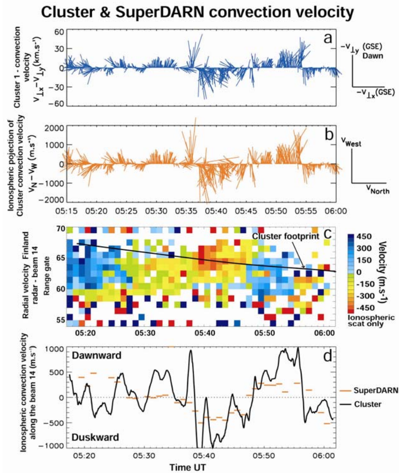
Fig. 4.6 : Evénement du 17/03/2001. Vitesses de convection mesurées par SuperDARN et Cluster-1. (a) Vecteurs vitesse perpendiculaire des ions (voir explication dans le commentaire de la figure 4.3). (b) Projection dans l'ionosphère à 250 km d'altitude des vecteurs vitesse de CIS, où V_{west} et V_{north} correspondent aux composantes de la vitesse dans les directions ouest et nord magnétique respectivement, en coordonnées AACGM. (c) Diagramme temps-distance de la vitesse radiale pour le faisceau 14 du radar d'Hankasalmi, avec superposée la projection de Cluster (ligne noire). (d) Comparaison des vitesses de convection mesurées par Cluster (ligne noire) et par SuperDARN (segments rouges). La vitesse de convection CIS a été moyennée sur 1 minute et projetée le long du faisceau 14 d'Hankasalmi. La vitesse SuperDARN est la vitesse radiale mesurée au pied de la ligne de champ de Cluster.
