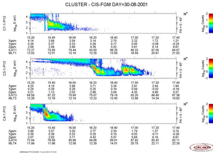
Fig. 5.7 : Evénement du 30/08/2001. Spectrogrammes des flux des ions H^+ en fonction du temps et de l'énergie, mesurés par Cluster-CIS et dans la direction parallèle au champ magnétique (angle d'attaque=0-40°), pour les satellites 1-3-4, sur la période 15:20-17:40 TU.
