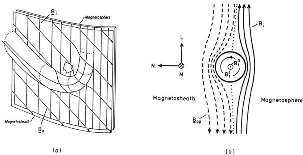
Fig. 2.1 : Schéma d'un FTE à la magnétopause. (a) dans un plan parallèle à la magnétopause. Les lignes verticales représentent le champ magnétosphérique et les lignes inclinées représentent le champ magnétique dans la magnétogaine. La flèche blanche montre la direction de la tension magnétique. (b) dans un plan perpendiculaire à la magnétopause. Le champ magnétique principal du tube de flux est suivant l'axe du tube B_i^0 , auquel s'ajoute un faible champ azimuthal B_i^1 créé par les courants alignés avec le champ (d'après Russel et Elphic, 1979).
