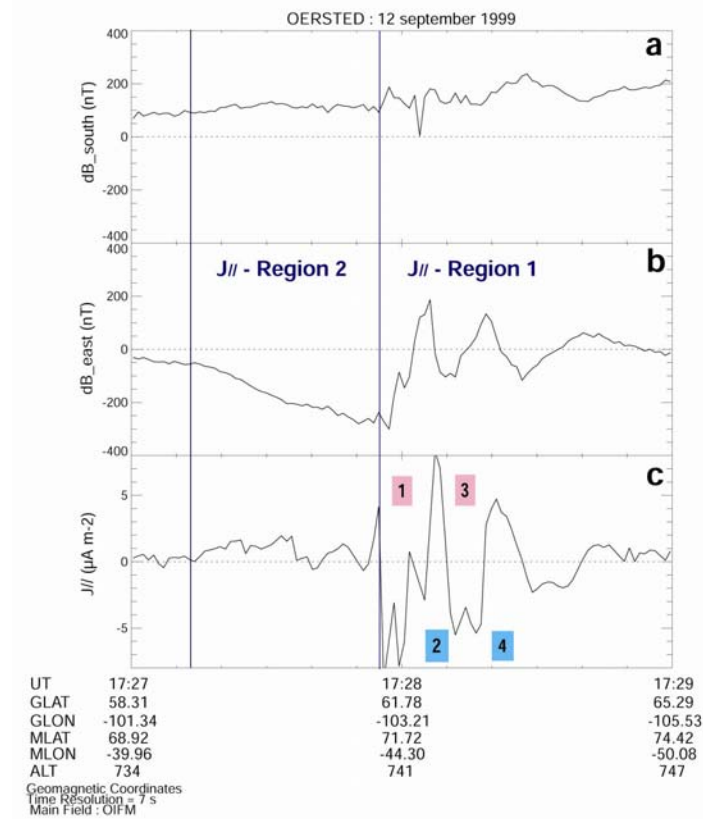
Fig. 7.4 : Evénement du 12 septembre 1999. (a) Champ magnétique et courants alignés mesurés par Ørsted. (a) Composante nord-sud. (b) Composante est-ouest. (c) Courants alignés moyennés sur 7 secondes. Les courants positifs correspondent aux courants montants et les courants négatifs correspondent aux courants descendants. Les lignes bleues délimitent les Régions -1 et -2 de courants parallèles à grande échelle. Les chiffres 1 à 4 correspondent aux 4 nappes de courants à petite échelle.
