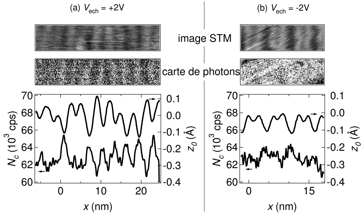
FIG. 4.4 – Emission induite par STM d’une surface de Au(111) pour (a) V_{\text{ech}} > 0 et (b) V_{\text{ech}} < 0 . En haut, sont représentées l’image STM et la carte de photons. En bas, les profils obtenus en moyennant les lignes de la topographie (trait plein) et celles de la carte de photons ( -\blacktriangle- ) sont tracées en fonction de x , désignant la direction, sur la surface, perpendiculaire aux lignes de reconstruction. Il existe un contraste net sur le nombre de photons émis pour V_{\text{ech}} > 0 , ce qui n’est pas le cas pour V_{\text{ech}} < 0 .
