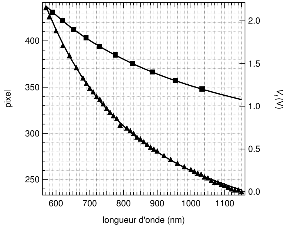
FIG. C.2 – Dispersion du spectromètre. Le numéro du pixel (origine absolue arbitraire) est représenté en fonction de la longueur d'onde (—▲—). Pour faciliter la conversion eV nm, la tension tunnel correspondant à la longueur d'onde est donnée —■—), les carrés représentant des valeurs typiques de tensions dans les conditions d'émission induite par STM.
