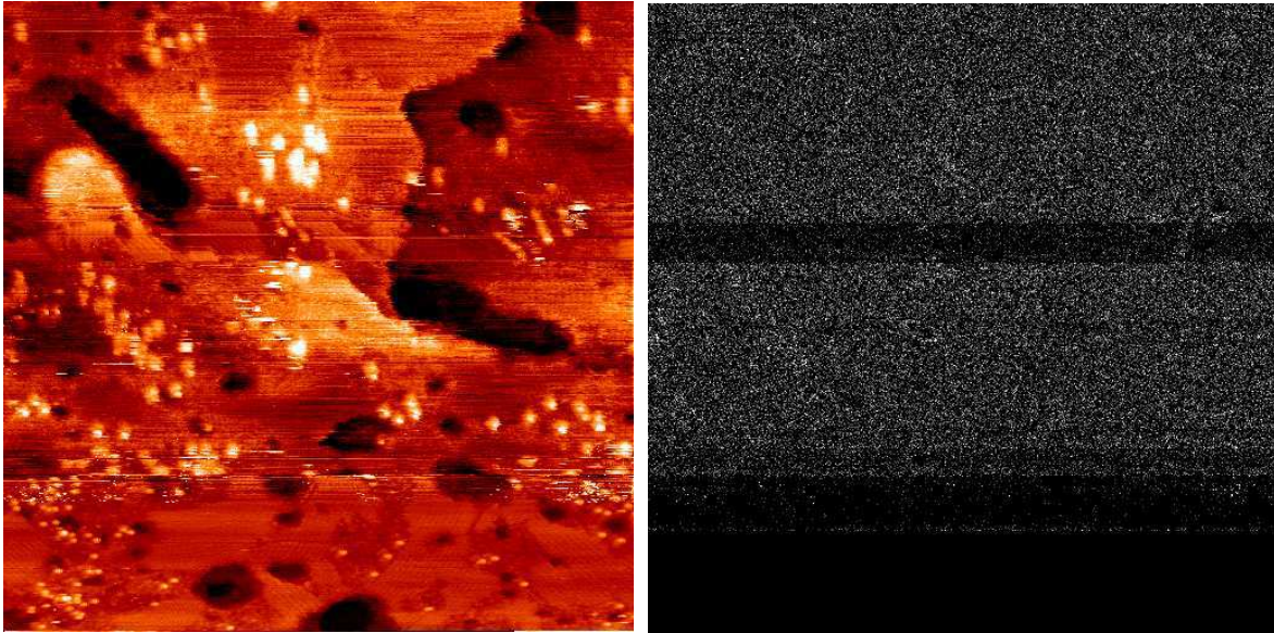
FIG. 8.15 – Emission de photons d'un système C_{60} sur OT sur Au(111) : modifications du rendement avec la pointe. L'image ( (100 \times 100) nm 2 , V_{\text{ech}} = -1,5 V, I_c = 1 nA, pointe en or) a été enregistrée en balayant de droite à gauche (direction de balayage rapide) et de bas en haut (direction de balayage lent). L'image de gauche représente la topographie et celle de droite, la carte de photons. En bas, V_{\text{ech}} = -0,4 V : la topographie est bien résolue, il n'y a pas d'émission. Ensuite, V_{\text{ech}} = -1,5 V : l'image est moins bien résolue, par contre, des photons sont détectés. Sans que les paramètres de l'image n'aient changé, on observe une bande sur la carte de photons où le niveau d'émission est beaucoup plus faible (quoique supérieur au bruit d'obscurité). En même temps, la résolution sur la topographie est meilleure. Une molécule de C_{60} est probablement adsorbée sous la pointe. Quand elle se désorbe, on retrouve le niveau d'émission et la résolution précédents.
