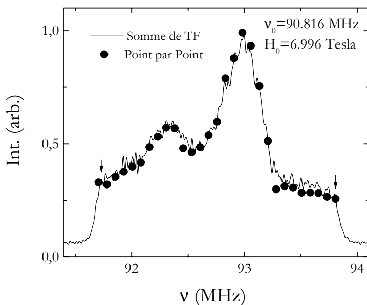
Figure II-9 : Spectre RMN de ^{71}\text{Ga} à T=150 K pour \text{SrCr}_p\text{Ga}_{12-9p}\text{O}_{19} ( p=.89 ) dans un champ fixe H_0=6.9955 Tesla avec la méthode point par point (cercles solides) et la méthode par somme de transformée de Fourier (trait plein). Les flèches indiquent une coupure artificielle liée à la technique par somme de transformée de Fourier.
