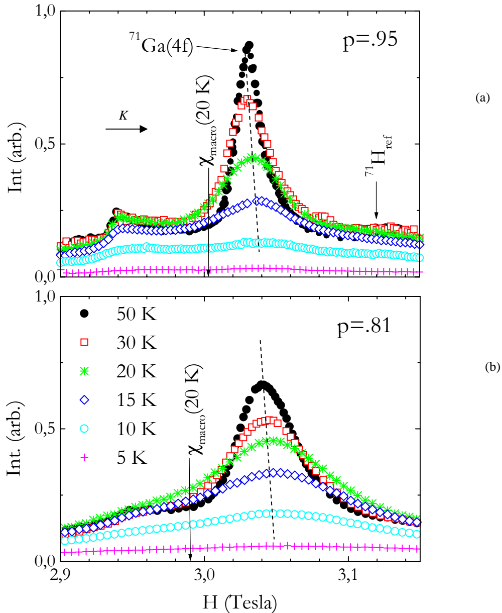
Figure V-2 : (a) Série de spectres de ^{71}\text{Ga}(4f) à \nu_{ij}=40.454 \text{ MHz} ( ^{71}\text{H}_{\text{ref}}=3.116 \text{ Tesla} ) pour l'échantillon p=0.95 . La droite en pointillés est une aide à la lecture. La structure quadrupolaire, qu'on peut encore apercevoir à T=50 \text{ K} , disparaît progressivement à température décroissante. La singularité à H \approx 2.94 \text{ Tesla} est celle de ^{71}\text{Ga}(4e)^{\text{RC}} . La flèche avec le label \chi_{\text{macro}}(20 \text{ K}) indique la position approximative où devrait se trouver le maximum de ^{71}\text{Ga}(4f) à T=20 \text{ K} si K \equiv \chi_{\text{macro}} . (b) Série de spectres de ^{71}\text{Ga}(4f) à \nu_{ij}=40.454 \text{ MHz} pour l'échantillon p=0.81 .
