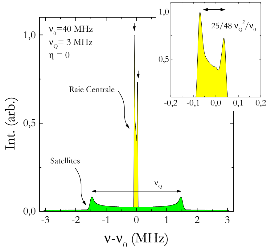
Figure II-5 : Spectre de poudre en présence d'effets quadrupolaires seuls, au 2 ème ordre en perturbation pour la raie centrale et au 1 er ordre pour les satellites. Dans une expérience de RMN par impulsion, l'intensité des satellites (aire intégrée) est proportionnelle à la racine carrée de l'intensité des transitions -1/2 \leftrightarrow 3/2 et 3/2 \leftrightarrow 1/2 , soit à I_{sat} = 2\sqrt{3} [Fukushima, 1981]. L'intensité de la raie centrale est proportionnelle à la racine carrée de la transition 1/2 \leftrightarrow 1/2 , soit à I_{RC} = \sqrt{4} . Le rapport des deux intensités est I_{sat}/I_{RC} = \sqrt{3} , donc 63% de l'intensité totale est dans les satellites et 37% dans la raie centrale. Encadré : Agrandissement de la raie centrale.
