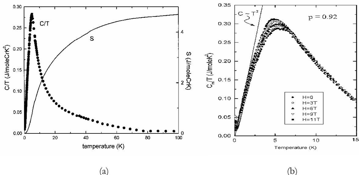
Figure I-13 : (a) Variation en température de la chaleur spécifique magnétique, divisée par la température, C(T, H)/T , pour \text{SrCr}_{9p}\text{Ga}_{12-9p}\text{O}_{19} , p=.89 . La ligne solide représente la chaleur spécifique intégrée, c'est-à-dire l'entropie [d'après Ramirez, 2000]; (b) Chaleur spécifique à plusieurs champs H pour \text{SrCr}_{9p}\text{Ga}_{12-9p}\text{O}_{19} , p=.92 [d'après Ramirez, 2000].
