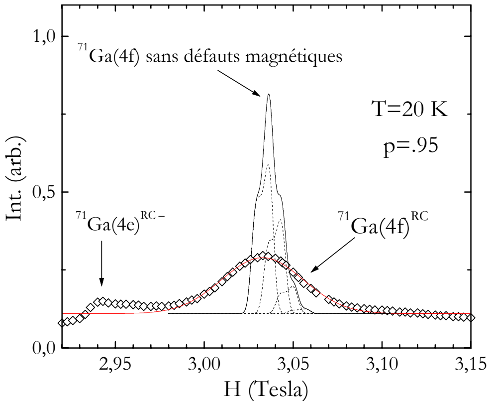
Figure VI-12 : Comparaison du spectre en balayage de champ de ^{71}\text{Ga}(4f) pour l'échantillon p=.95 obtenu à T=20\text{ K} avec la forme de raie attendue s'il n'existait pas de défauts magnétiques dans la bi-couche kagomé. Les aires de la raie expérimentale et de la raie simulée sont normalisées. L'aire de la raie expérimentale a été évaluée avec un ajustement gaussien (trait plein) et est connue à 10% près. Le déplacement de la raie simulée est égal à celui de la raie expérimentale.
