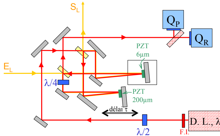
FIG. 2.47 – Montage expérimental partiel du « \chi^{(2)} portable» (Chideuportatif) version deux impulsions (voir texte). E_L et S_L sont respectivement l'entrée et la sortie du laser exciteur. D.L. est la diode laser à la longueur d'onde \lambda qui stabilise le montage suivant le principe de la figure 2.20. Q_P et Q_R sont des photodiodes qui détectent des franges temporelles de même nom. Devant chacune est placé un polariseur. Les lames retard demi-onde ( \lambda/2 ) et quart d'onde ( \lambda/4 ) modifient la polarisation de la diode mais pas celle du laser L. PZT : cales piézoélectriques de course 6 \mu\text{m} ou 200 \mu\text{m} . FI : filtre interférentiel.
