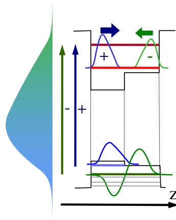
FIG. 3.39 – Représentation schématique de l'interférence entre deux paquets d'ondes électroniques issus de l'excitation de deux sous-bandes de valence différentes par une impulsion large-bande.
