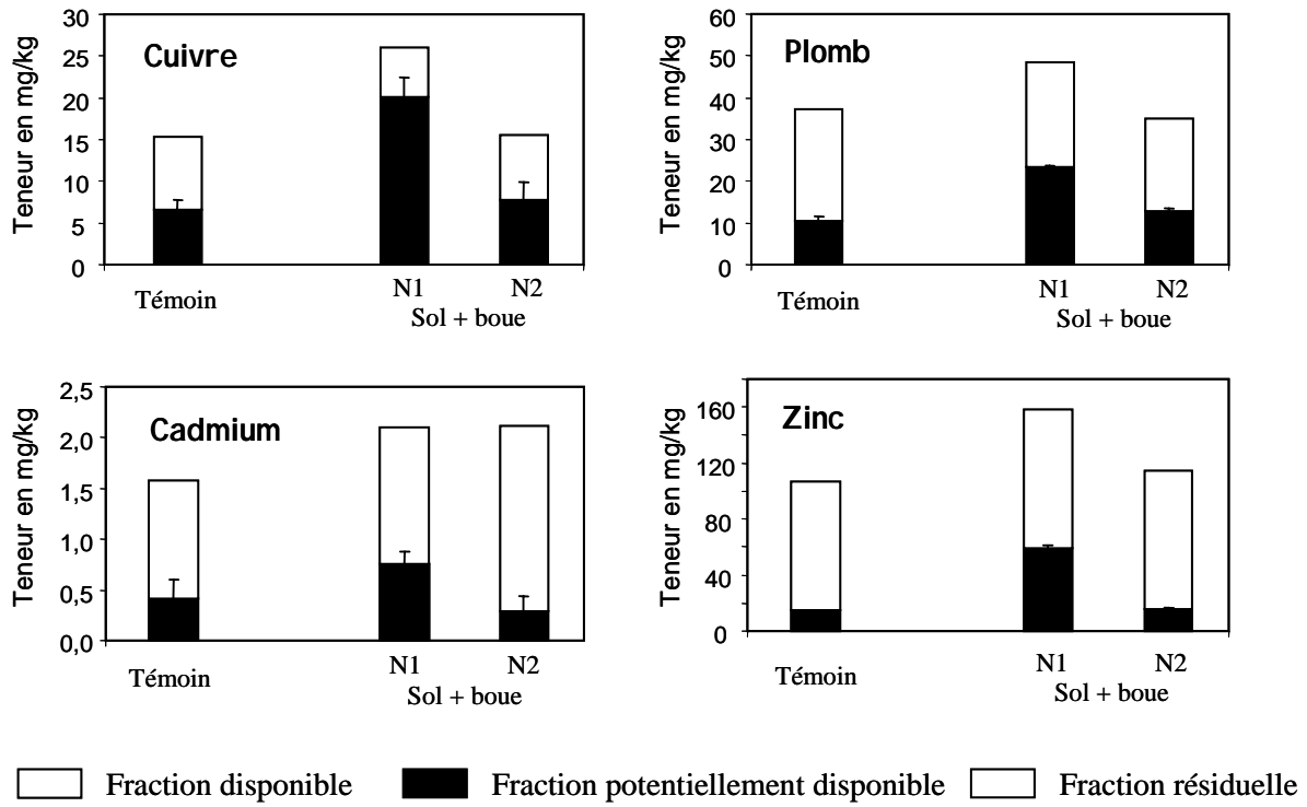
Figure IV.7 Teneurs en ETM dans les fractions résiduelle, potentiellement disponible, disponible du sol des modalités Témoin et Boue.
