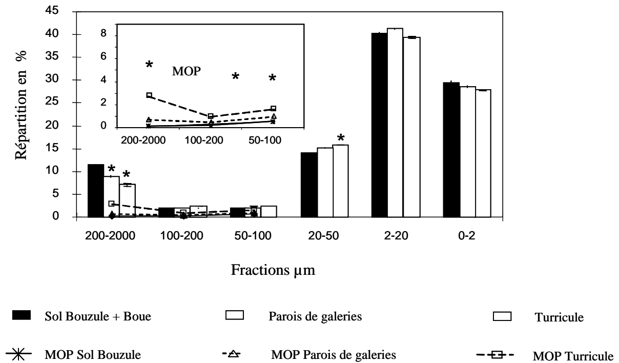
Figure IV.14 Granulométrie des turricules et parois de galeries de N. giardi
