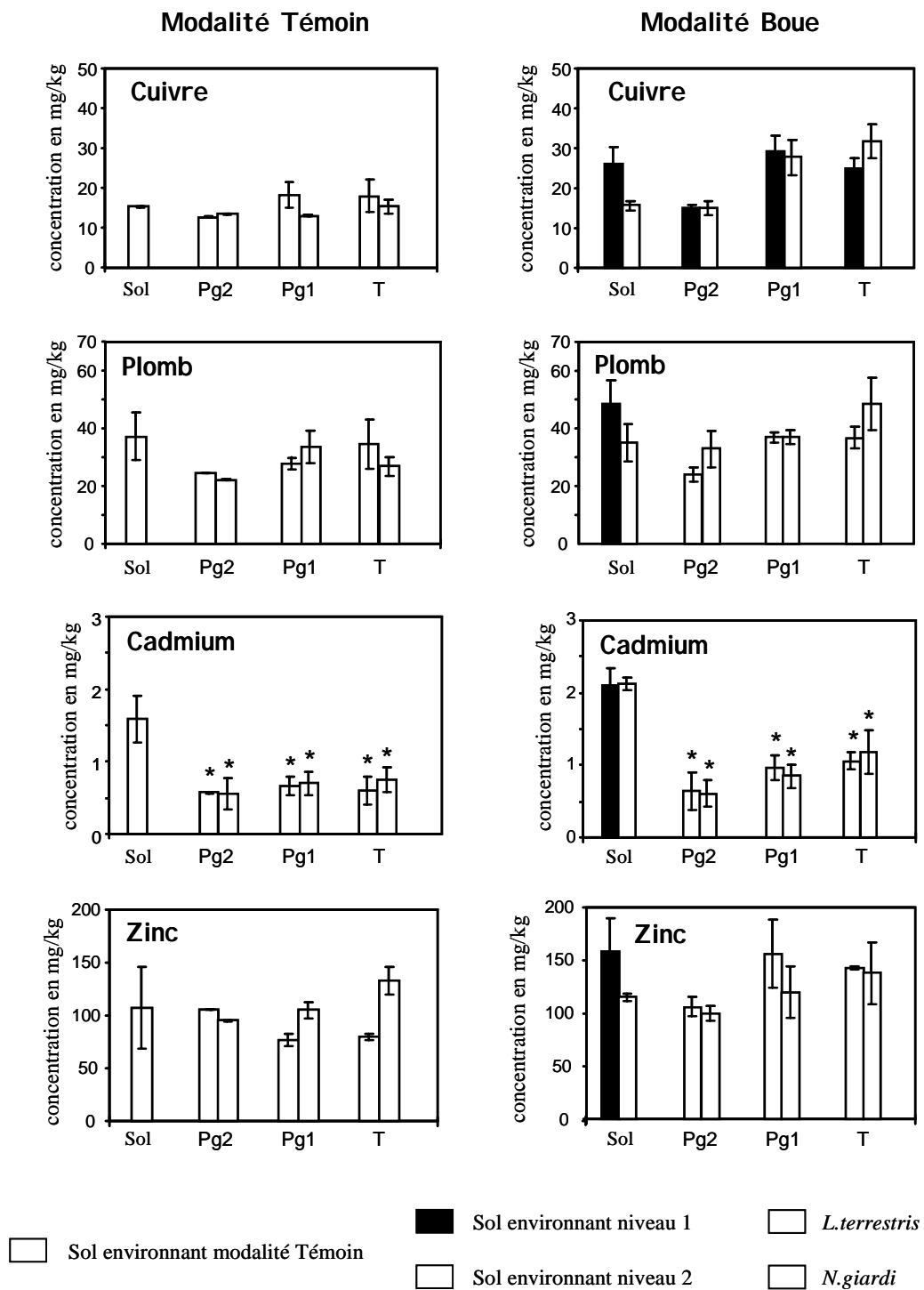
Figure IV.4 Tenures totales en ETM dans le sol environnant, les parois de galeries et les turricules de L.terrestris et N.giardii pour les modalités Témoin et Boue.
