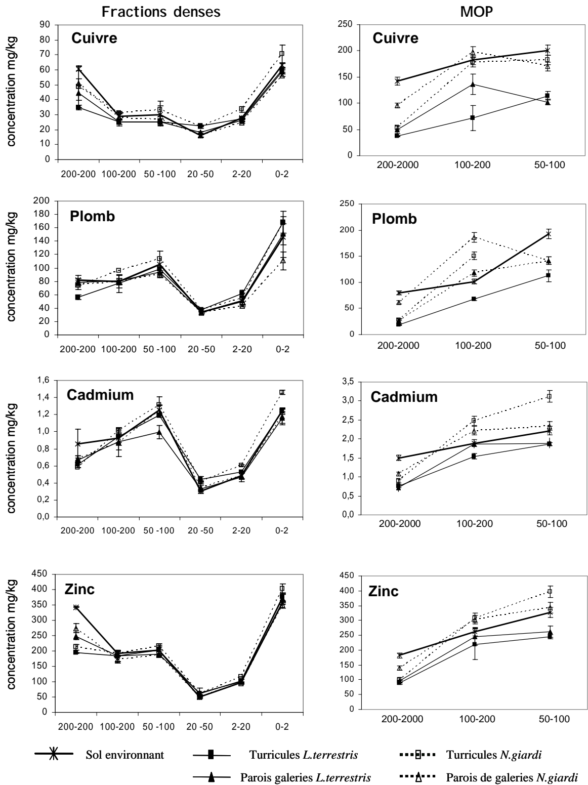
Figure IV.18 Concentration en ETM dans les fractions granulo-densimétriques du sol environnant, des parois de galeries et des turrucules de L. terrestris et N. giardi .
