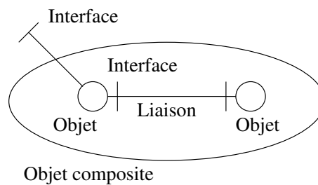
FIG. 2.14 – Modèle de composants RM-ODP
