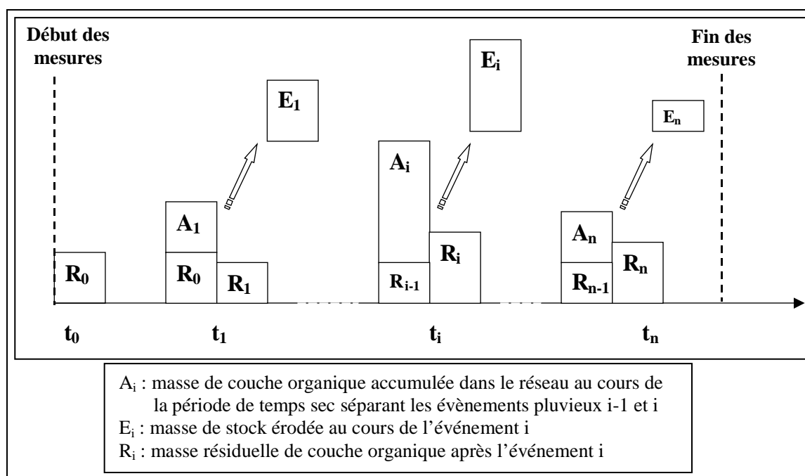
Figure IV-11 – Schéma conceptuel de l'érosion de la couche organique (Ahyerre, 1999)
