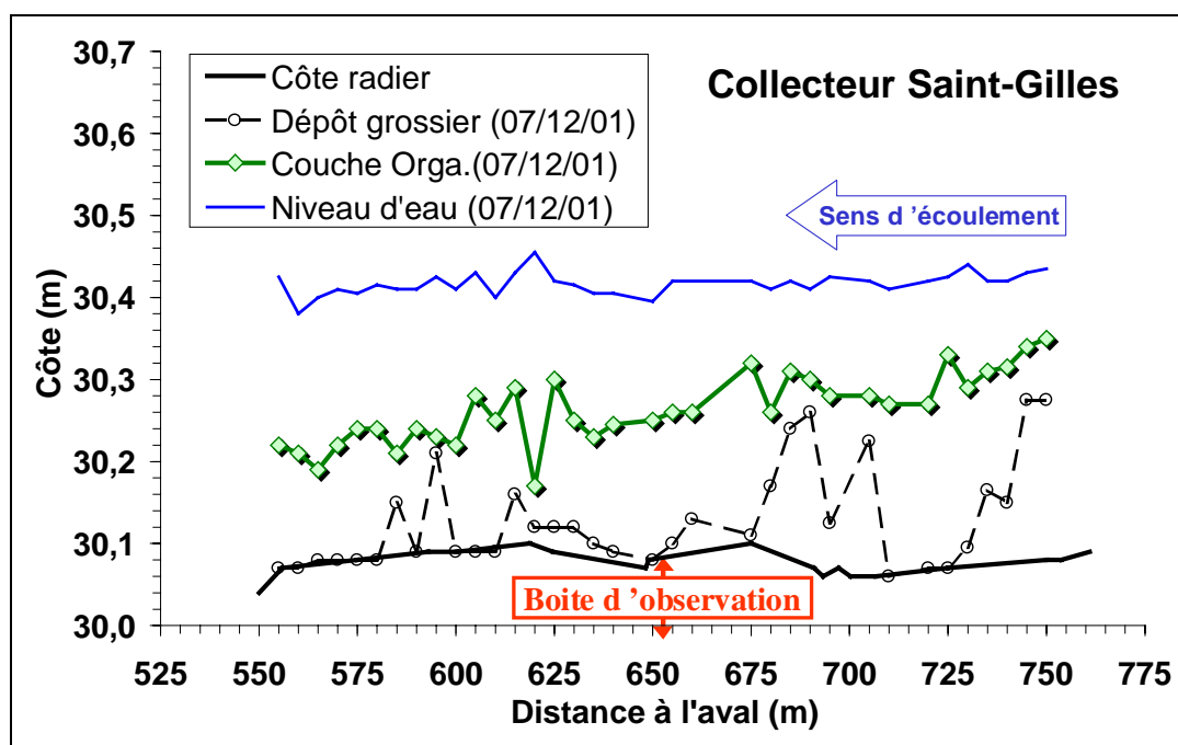
Figure IV-15 – Etat du collecteur étudié en décembre 2001
