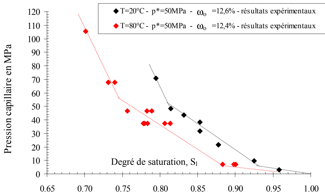
Figure I.29. : Isothermes capillaires à 20°C et à 80°C de l'argile FoCa 7 compactée avec une pression p^* de 50 MPa et une teneur en eau d'environ 12.5 %. Résultats expérimentaux et linéarisations (en pointillé).
