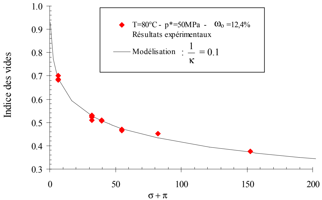
Figure 1.33. : Valeur du coefficient ( 1/K ) à 80^{\circ}\text{C} pour l'argile FoCa 7 compactée avec une pression de 50 MPa et une teneur en eau de 12.4 %..
