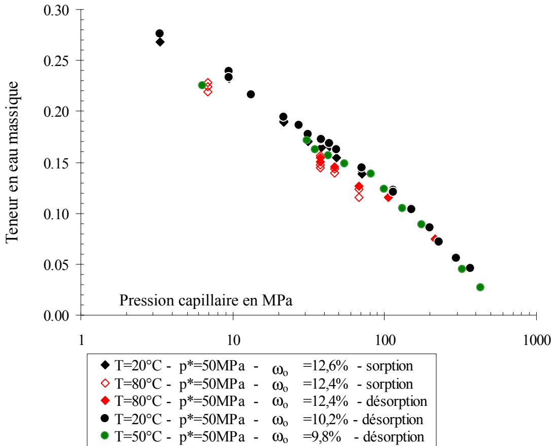
Figure I.23. : Influence de la température sur le comportement hydrique à volume libre.
