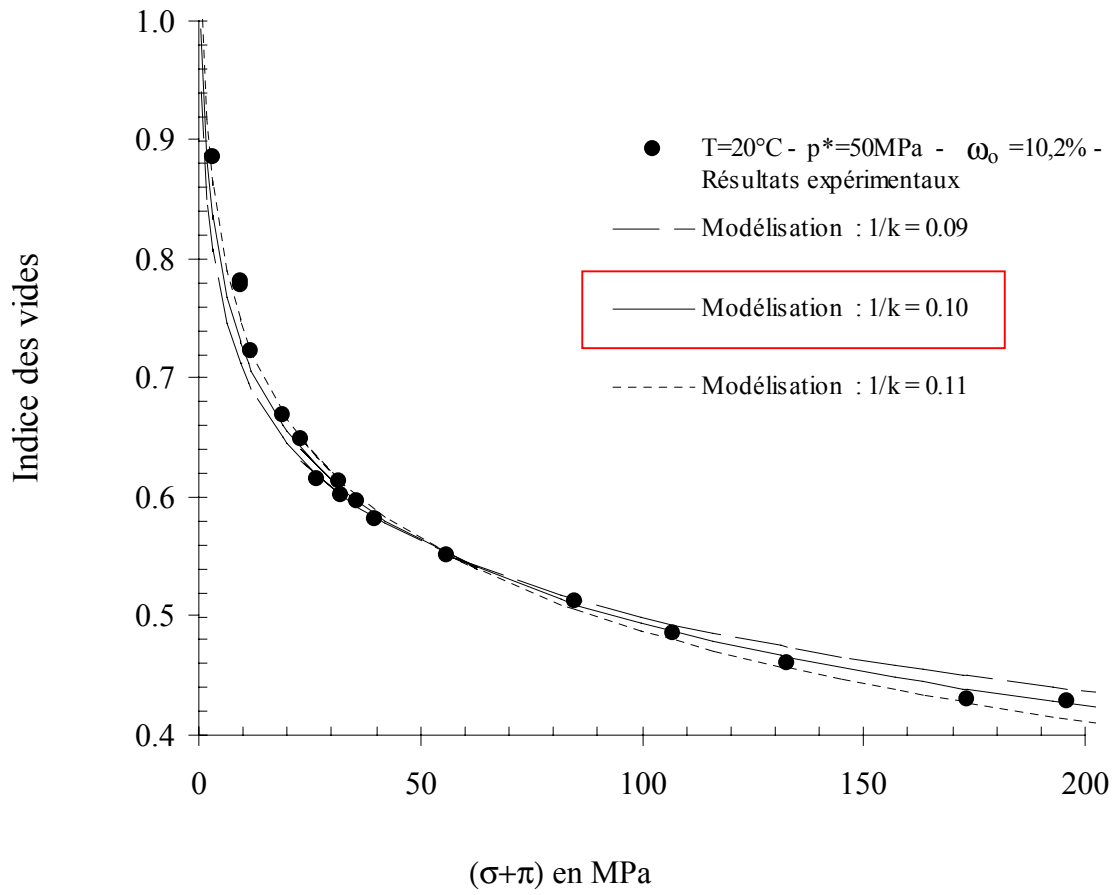
Figure I.30. : Valeur du coefficient (1/K) à 20°C pour l'argile FoCa 7 compactée avec une pression de 50 MPa et une teneur en eau de 10.2 %.
