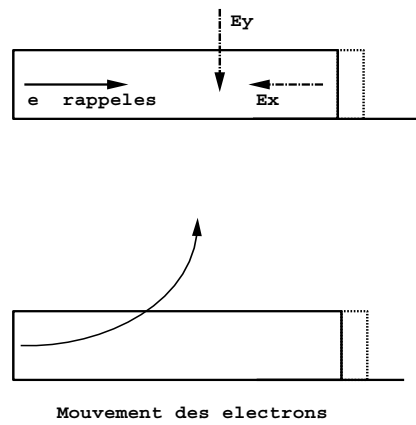
FIG. 2.3 – Pompage
