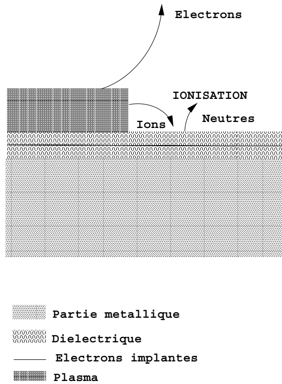
FIG. 1.1 – Principe de la décharge
