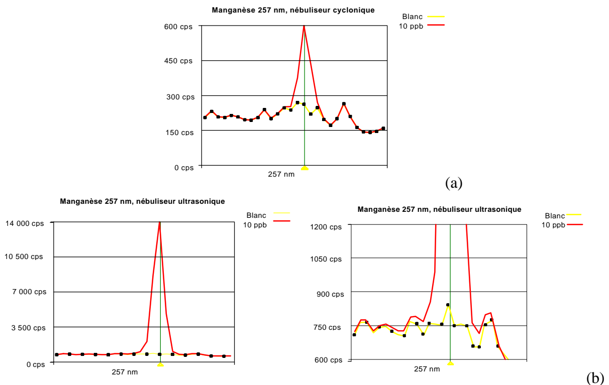
Figure II-10: Pics d'émission de Mn pour une même concentration dans le cas d'une analyse par ICP-AES comprenant un nébuleur Meinhart (a) et un nébuleur ultrasonique (b).
