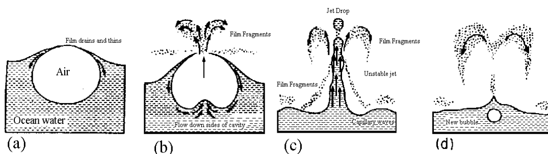
Figure A I-1: La production des sels de mer se fait selon quatre étapes suite au pétillage océanique. (a) La bulle d'air arrive à la surface de l'océan et seule une fine couche d'eau marque l'interface entre la bulle et l'atmosphère. (b) la bulle éclate en dispersant dans l'air le film d'eau restant. (c) le flux d'eau crée lors de l'éclatement de la goutte entraîne un petit jet d'eau libérant des gouttes d'eau dans l'atmosphère. (d) les particules de sel restent dans l'air une fois la goutte d'eau évaporée (Pruppacher & Klett, 1997).
