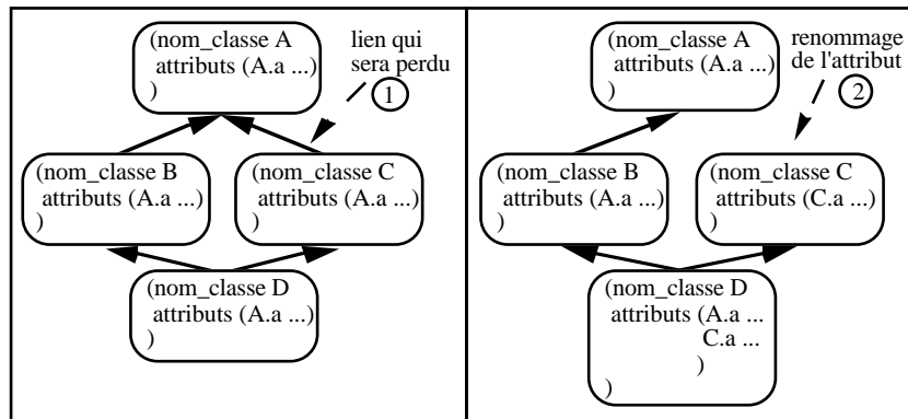
Figure 2.17. Le renommage de l'attribut A.a dans la classe C produit une partition de l'attribut en question dans la classe D.
