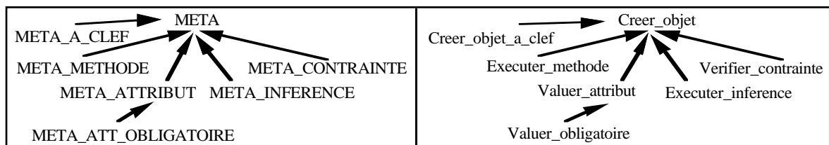
Figure 4.18. Graphe des méta-classes et de ses méthodes associées du graphe Creer_objet .
