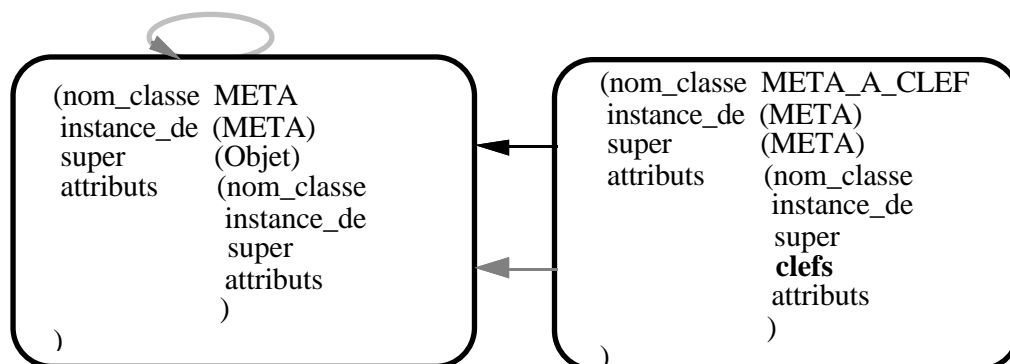
Figure 4.3. Premier pas dans la définition des classes à clef
