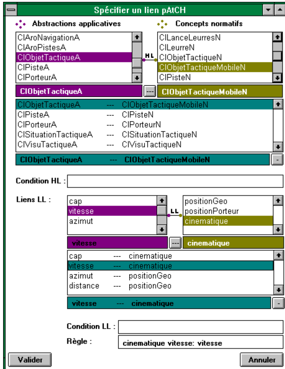
Figure 105 : Fenêtre de spécification des liens pAtCH.
