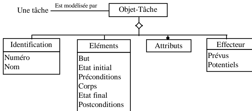
Figure 68 : Modélisation OMT des tâches de CoTaS.
