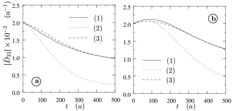
Fig. 5.4 : Evolution de la valeur absolue de la vitesse de déformation dans la direction e_3 en fonction du temps t pour |\bar{S}_{33}| = 0.1 \text{MPa} et B_1 = 0.04 \text{MPa}^{-1} \text{a}^{-1} en (a) traction uniaxiale et (b) compression uniaxiale. Courbe (1) : modèle SC1, pour \beta = 0.04 et \psi = 0.4 ; courbe (2) : modèle à contraintes homogènes pour \beta = 0.04 et \psi = 0.094 ; courbe (3) : modèle à contraintes homogènes pour \beta = 0.25 et \psi = 0.073 . La valeur \beta = 0.04 correspond à \psi/B_1 = 10 pour le modèle SC1.
