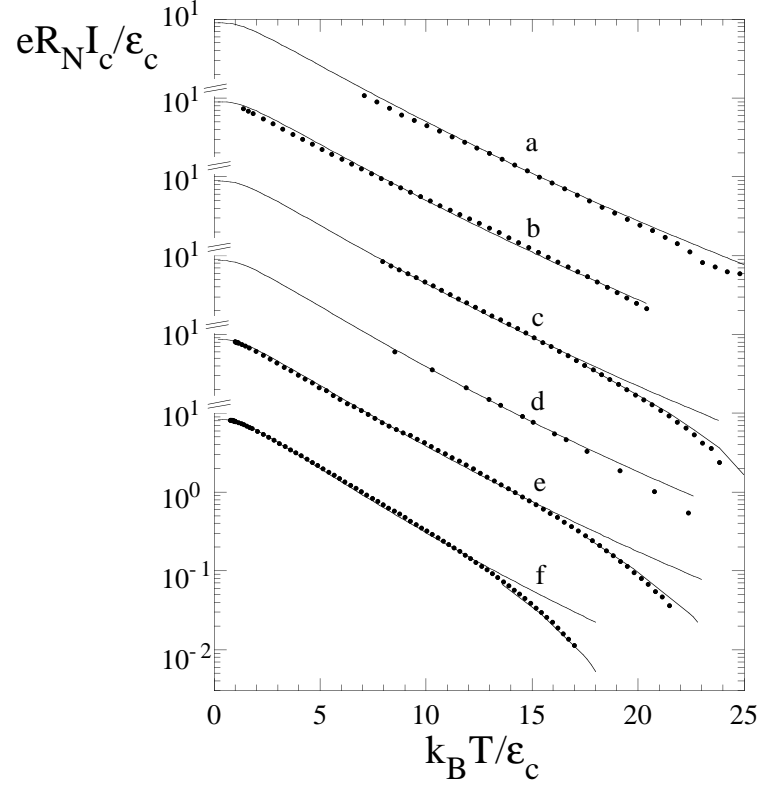
FIG. 3.11 – Courant critique eR_N I_c des six échantillons en fonction de la température. Les unités sont normalisées à l'énergie de Thouless \epsilon_c de chacune des jonctions. Les lignes continues représentent les courbes théoriques pour un gap indépendant de la température. Un meilleur accord est obtenu à haute température en tenant compte de la fermeture du gap suivant la théorie BCS pour une température critique T_c = 7.5 K. La liste des paramètres est présentée au tableau 3.1.
