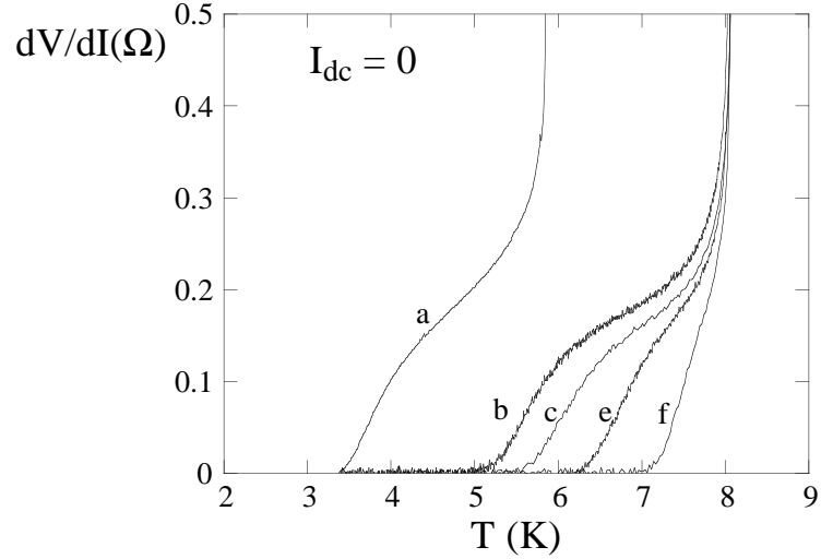
FIG. 3.8 – Mesure de la résistance différentielle en fonction de la température pour les échantillons (a, b, c, e, f). Le courant de polarisation I_{dc} = 0 . La température critique du niobium vaut T_c = 6 K pour l'échantillon (a) et T_c = 8.1 K pour les jonctions (b, c, d, e, f).
