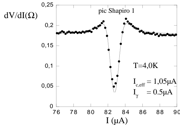
FIG. 5.4 – Ajustement de la dérivée de l'équation de Bishop et Trullinger (1.19) sur le pic Shapiro mesurés en V_1 à T = 4,0 K. La largeur effective vaut I_{c,eff}^1 = 1.05 \pm 0.02 \mu A .
