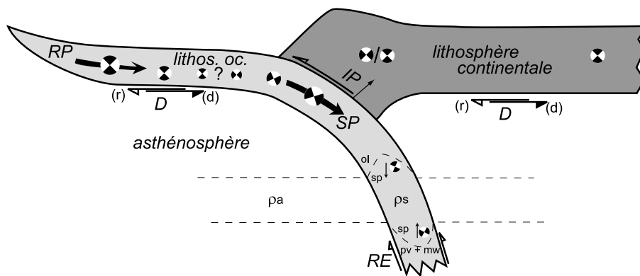
FIG. 1.2.3 – Schéma des forces principales agissant sur une zone de subduction. RP : poussée depuis la rive. SP : traction du panneau plongeant, ol (olivine), sp (spinelle) et pv + mw (perovskite+magnétowüsite) sont les phases (et les densités) du panneau plongeant. D : la friction à la base de la lithosphère. Elle peut être motrice (d) ou résistante (r), RE : résistance de l'asthénosphère à la pénétration du panneau plongeant. IP est la friction interplaque, c'est-à-dire la force transmise à la plaque chevauchante (d'après Forsyth et Uyeda, 1975, Chapple et Tullis, 1977). Les "ballons de plage" indiquent le régime tectonique présumé selon la convention habituelle.
