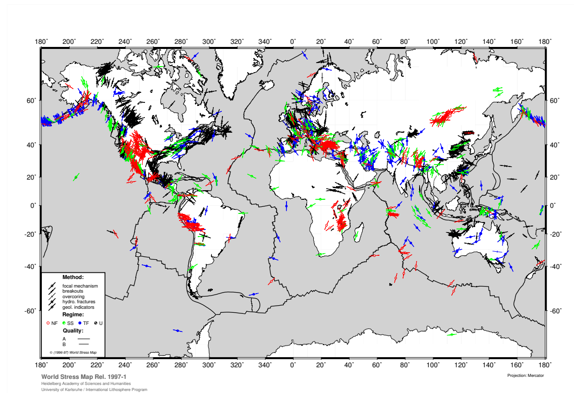
FIG. 1.2.2 – Carte globale des contraintes (d'après le World Stress Map Project, Mueller et al., 2000). Rouge : failles normales, vert : décrochements, bleu : failles inverses, noir : indéterminé. L'orientation donne la direction de contrainte horizontale maximale.
