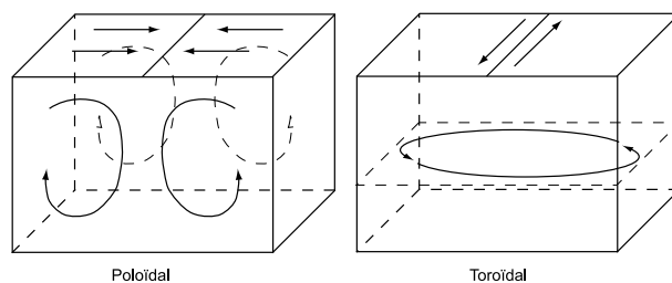
FIG. 3.3.13 – Description sch matique des composantes poloïdale et toroïdale.
