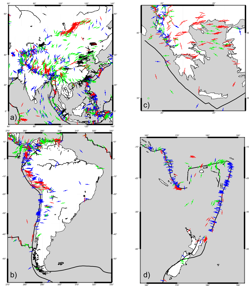
FIG. 1.2.6 – Régime de contraintes sur différentes zones de convergence. a) continent/ continent : SE Asie ; b) océan/ continent : Amérique du Sud ; c) océan/ continent : mer Egée ; d) océan/océan : Tonga-Kermadec (d'après les données de Mueller et al., 2000). Rouge : failles normales, vert : décrochements, bleu : failles inverses, noir : indéterminé. L'orientation donne la direction de la contrainte horizontale maximale.
