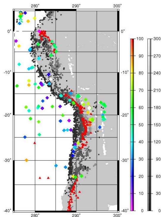
FIG. 1.5.11 – Sismicité profonde ( >50 km, en gris), volcanisme (triangles rouges) et flux de chaleur (losanges) dans les Andes. Le volcanisme souligne les segments où le panneau plongeant est penté, en corrélation avec la sismicité.
