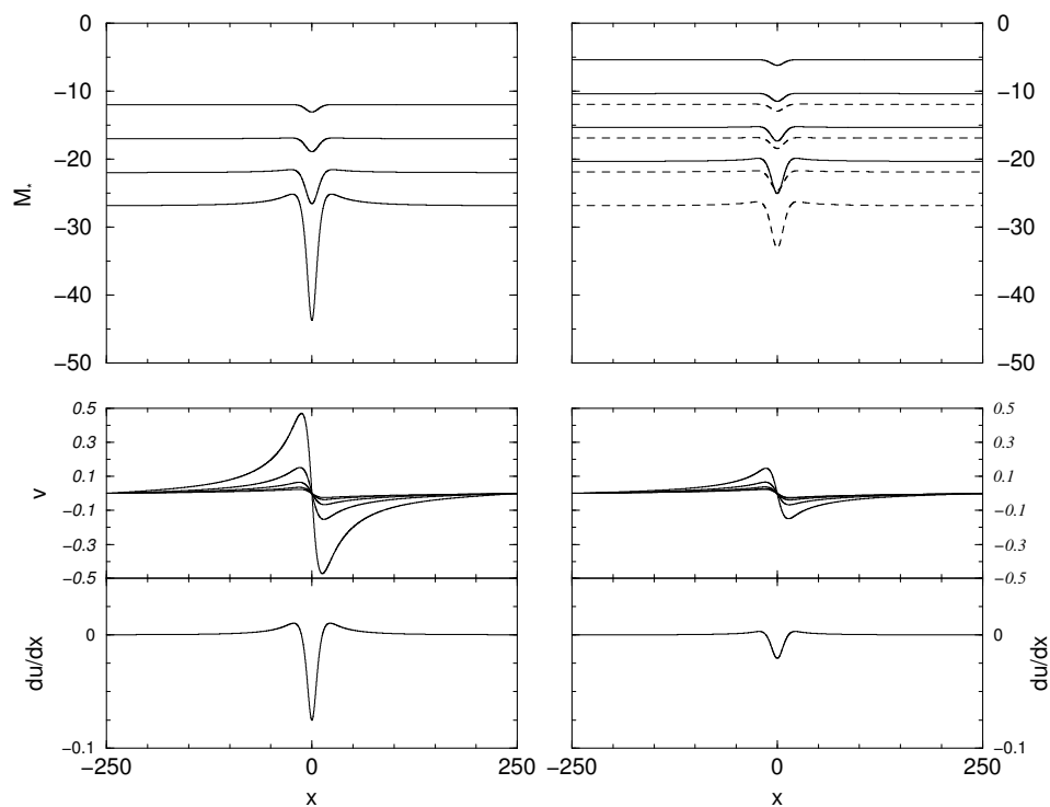
FIG. 3.4.18 – Evolution temporelle du moment lithosphérique total M (= M_C + M_L) et du champ de vitesse v , sans croûte (à gauche) et avec croûte (à droite). Les courbes tiretées donnent l'évolution du moment thermique seul. En l'absence de croûte, moment thermique M_L et moment total M sont confondus. Lorsque du/dx est négatif, le régime tectonique est compressif. Les grandeurs sont sans dimension.
