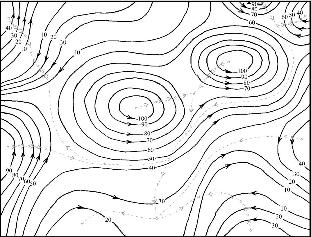
Carte isoplèthe et son graphe d'adjacence
