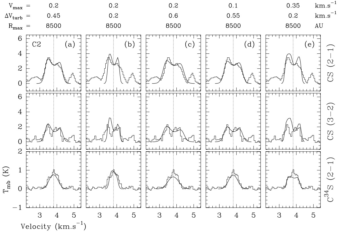
FIG. 5.11 – Effets de la dispersion de vitesse turbulente \Delta V_{\text{turb}} et de la vitesse maximale V_{\max} du champ de vitesse de contraction sur les spectres centraux CS(2-1) (1 ère ligne), CS(3-2) (2 ème ligne) et C 34 S(2-1) (3 ème ligne) de OphC-MM5. La colonne (a) rappelle le modèle C2 de la Fig. 5.5.
