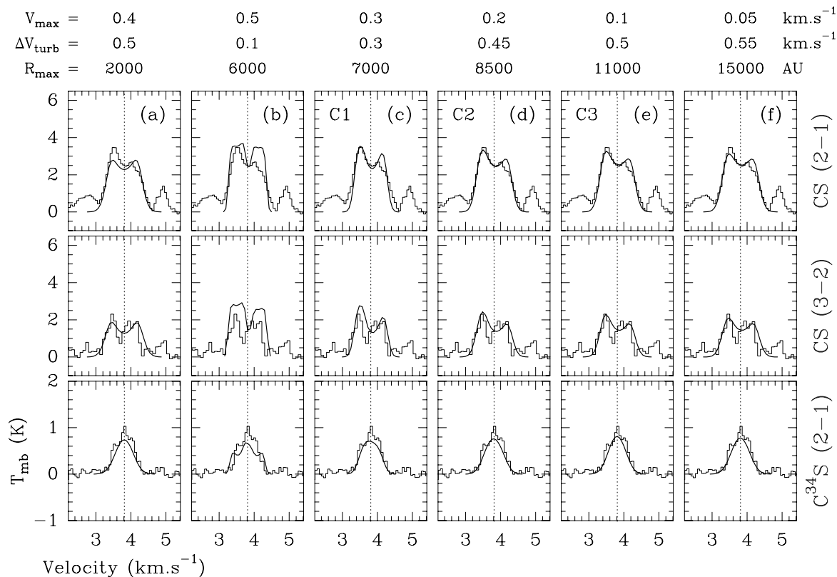
FIG. 5.12 – Effets du rayon R_{\max} et de la vitesse V_{\max} du pic de vitesse sur les spectres centraux CS(2-1) (1 ère ligne), CS(3-2) (2 ème ligne) et C^{34}\text{S}(2-1) (3 ème ligne) de OphC-MM5. Les colonnes (c), (d) et (e) rappellent les modèles C1, C2 et C3 des Fig. 5.4, 5.5 et 5.6.
