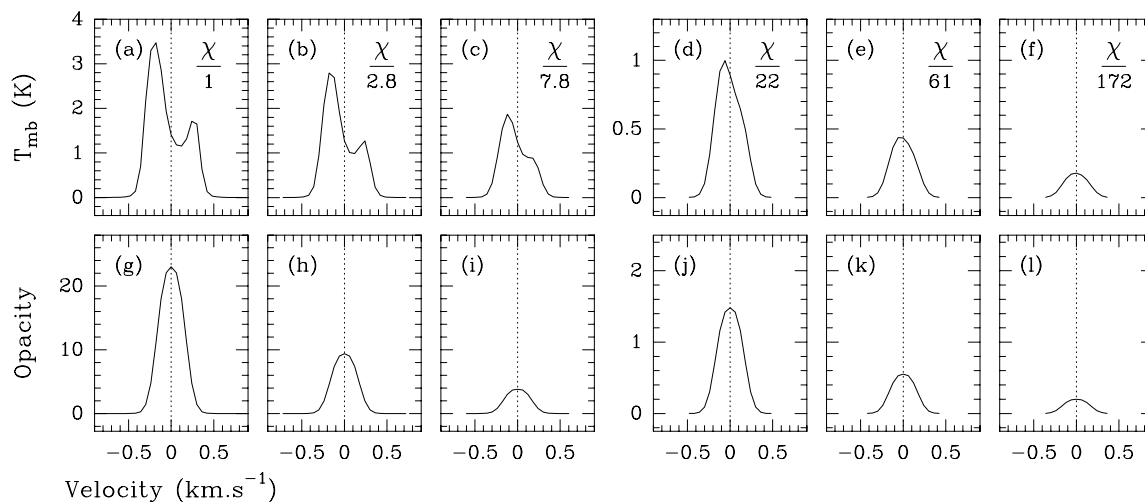
FIG. 3.4 – Variations de la signature spectroscopique d’effondrement avec l’opacité. Les graphiques (a) à (f) montrent l’évolution d’un spectre CS(2-1) pour une abondance variant de \chi (a) à \frac{\chi}{172} (f). Le spectre (a) est issu du modèle 1D d’enveloppe en effondrement réalisé pour IRAM 04191. Les profils d’opacité (g) à (l) montrent que la raie devient optiquement mince à partir du spectre (e). Le profil du spectre varie d’un profil asymétrique et auto-absorbé (a) vers un profil asymétrique avec seulement un épaulement du côté “rouge” (c), puis vers un profil symétrique (e) dès que l’opacité tombe en dessous de 1.
