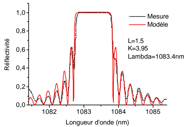
Figure D-2 : Miroir Rmax. Ajustement des paramètres du modèle vis-à-vis de la réflectivité mesurée.
