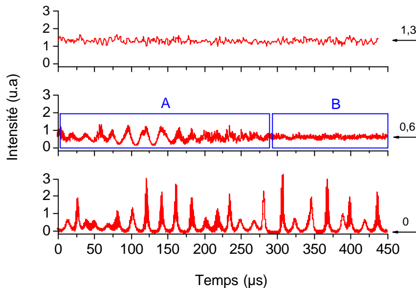
Figure III-26 : Traces temporelles des trois régimes de fonctionnement identifiés : En haut nous avons le régime stable Au centre le régime intermittent A étant une oscillation de relaxation et B un retour au régime stable En bas, le régime instable
