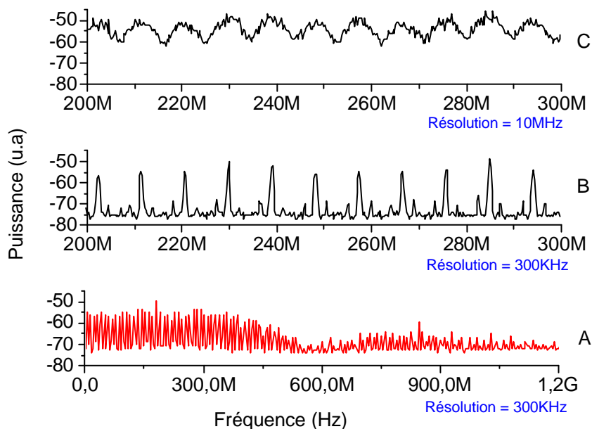
Figure III-25 : Laser à 1083 nm – Spectre basse fréquence Spectre C : 200 à 300 MHz - Résolution 10 MHz Spectre B : 200 à 300 MHz – Résolution 300 KHz (Agrandissement du spectre A) Spectre A : 0 à 1200 MHz – Résolution 300 KHz
