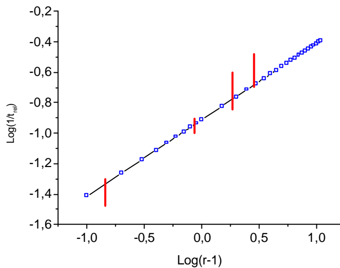
Figure III-38 : Périodes des oscillations de relaxation en fonction du taux de pompage pour R_{min} = 80\% et Pertes aux soudures simple passage = 10 % Symboles et trait continu : Relation 3-33 Traits verticaux : Résultats pour les 4 puissances de pompe de la figure III-37
