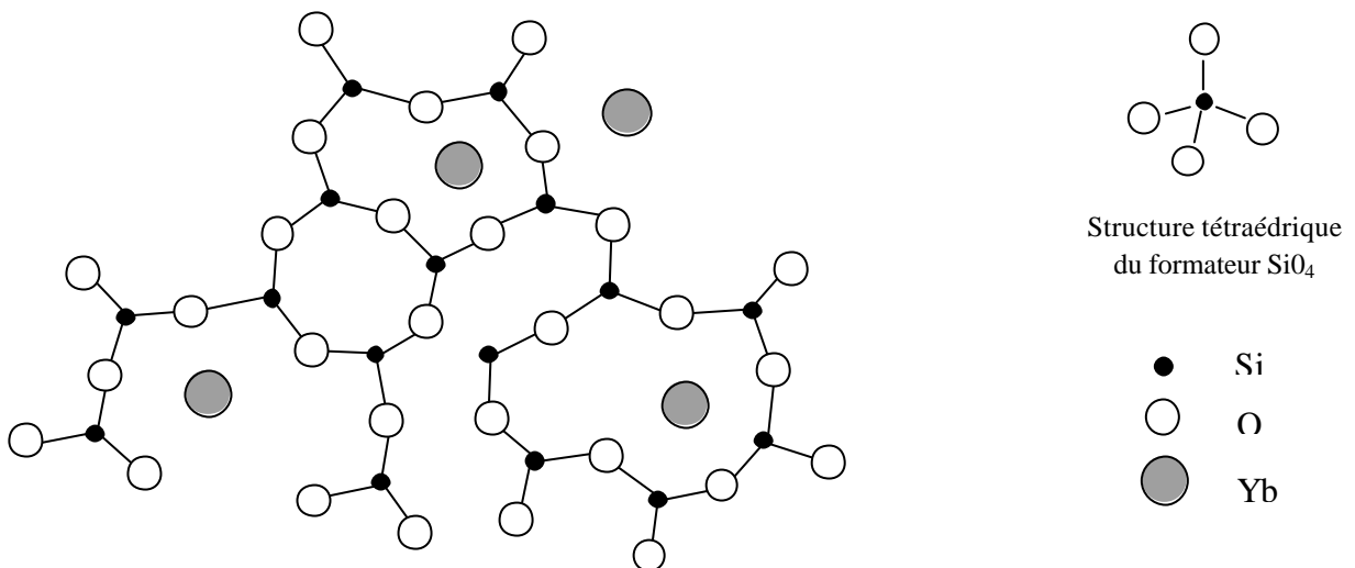
Diagramme II-3 : Représentation à 2 dimensions de la structure d'un verre de type silicate dopé Yb
