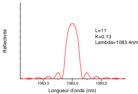
Figure D-3 : Miroir Rmin. Ajustement des paramètres du modèle pour obtenir la réflectivité et la largeur donnée par le fournisseur.
