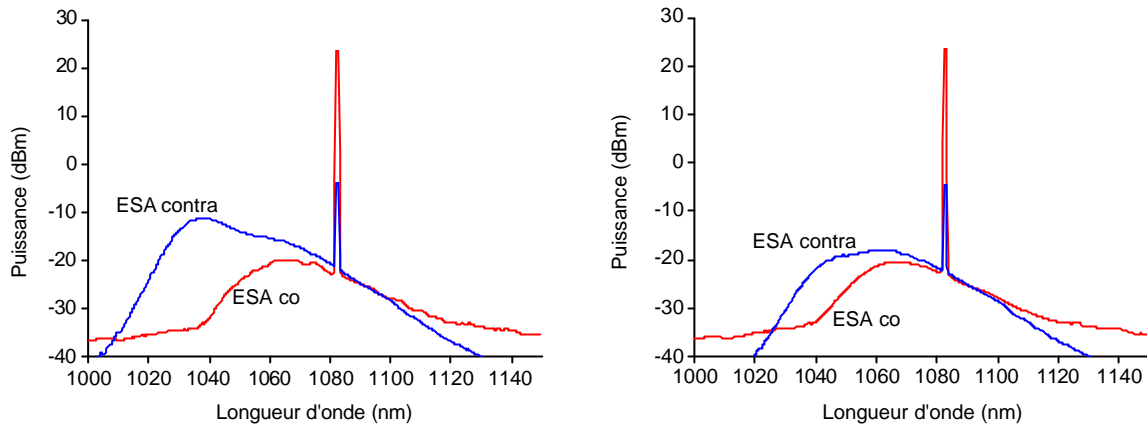
Figure III-15 : Spectre de sortie mesuré en C (ESA co) et en A (ESA contra) (Rés 0,25 nm). A gauche : Configuration de pompage co-propagatif. A droite : Configuration de pompage contra-propagatif.
