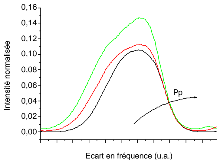
Figure III-20 : Laser à 1083 nm – Largeur de l'enveloppe spectrale en fonction de la puissance de pompe injectée R_{min} = X3 \% / Y1 \text{ pm} - P_p \text{ varie de } 0,68 \text{ W à } 1 \text{ W}
