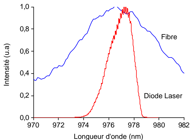
Figure III-3 : Position et largeur respective du spectre d'émission de la diode et de la bande d'absorption de la fibre 1. I = 3,5 \text{ A } T = 23 \text{ °C}
