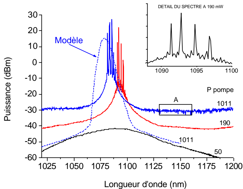
Figure III-46 : Laser en anneau – Spectre mesuré pour trois puissances de pompe (50, 190 et 1011 mW) (Rés 1 nm)
