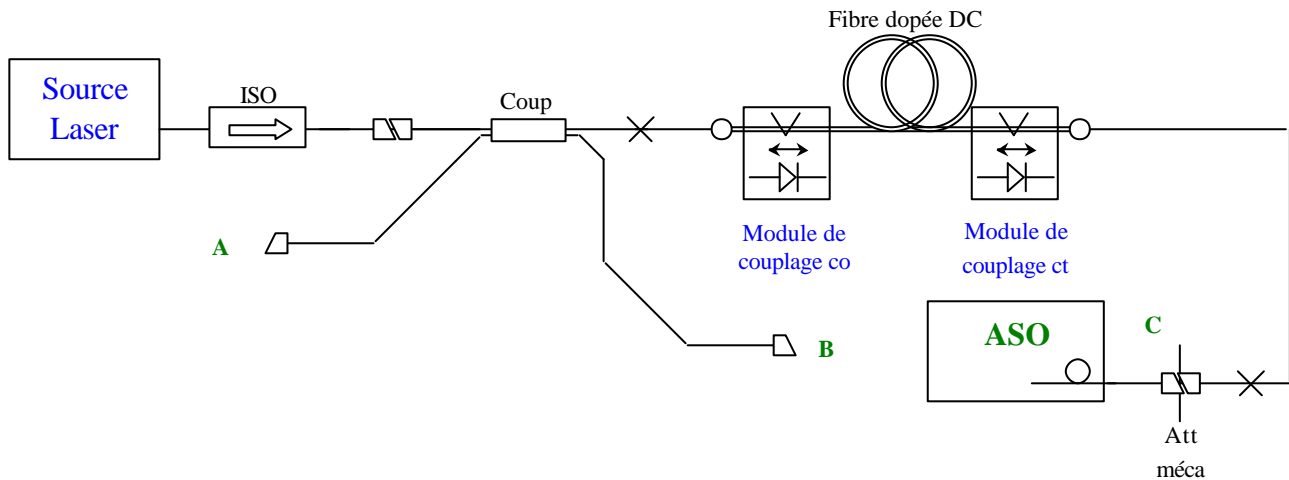
Figure III-24 : Schéma expérimental de caractérisation.
