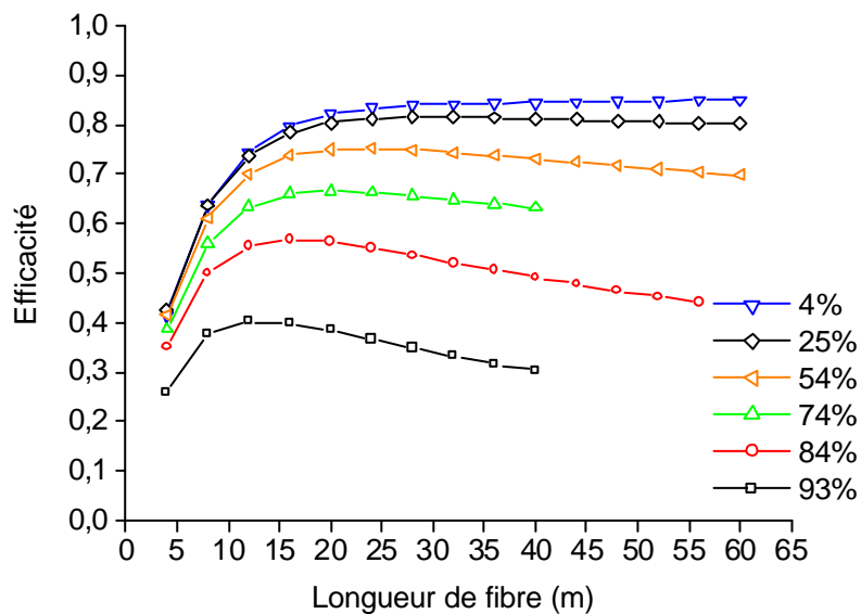
Figure III-11 : Laser à 1083 nm - Efficacité en fonction de la longueur de fibre dopée pour plusieurs réfectivités R_{min} . Pompage co -propagatif et pertes 1\%+1\% .
