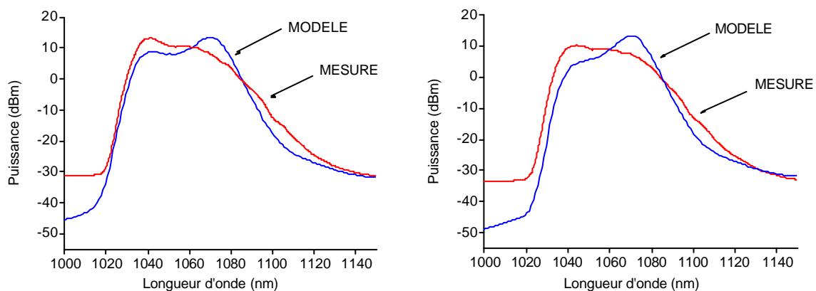
Figure III-20 : Comparaison des spectres de sortie mesurés avec le modèle (Rés 1 nm). A gauche : Configuration contra. A droite : Configuration co.
