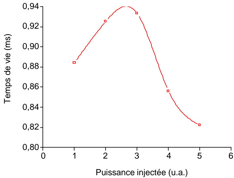
Figure III-2 : Variation du temps de vie mesuré avec la puissance de pompe injectée.
