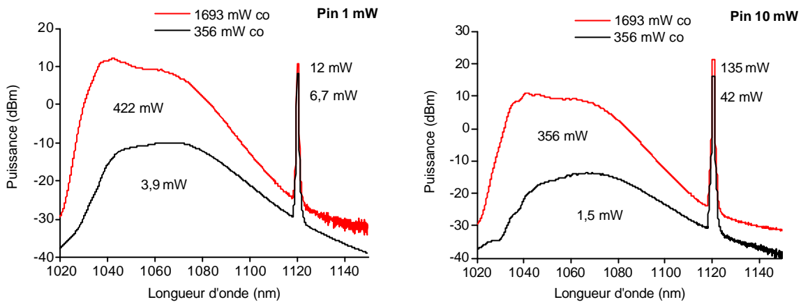
Figure III-49: Spectres mesurés pour deux puissances d'entrée (1 et 10 mW), et deux puissances de pompe injectées (1693 mW et 356 mW) (Rés 0,075 nm).
