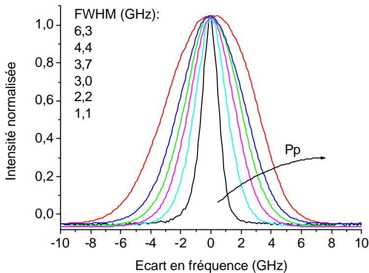
Figure III-19 : Laser à 1083 nm – Largeur de l’enveloppe spectrale en fonction de la puissance de pompe injectée. Rmin = X3 % / Y1 pm - Pp varie de 50 à 500 mW.
