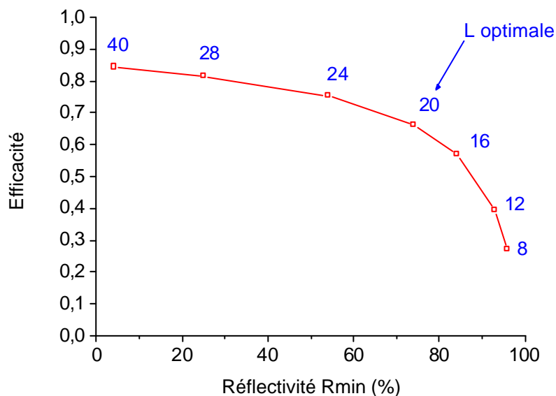
Figure III-13 : Laser à 1083 nm - Efficacité en fonction de la réflectivité du miroir Rmin Les pertes mesurées en B et D sont de 1 % + 1 % Pompage co - Longueur optimale donnée pour chacun des points.
