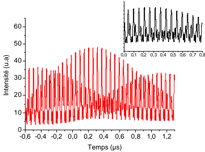
Figure III-41 : Détail d'une sous-séquence d'impulsion
