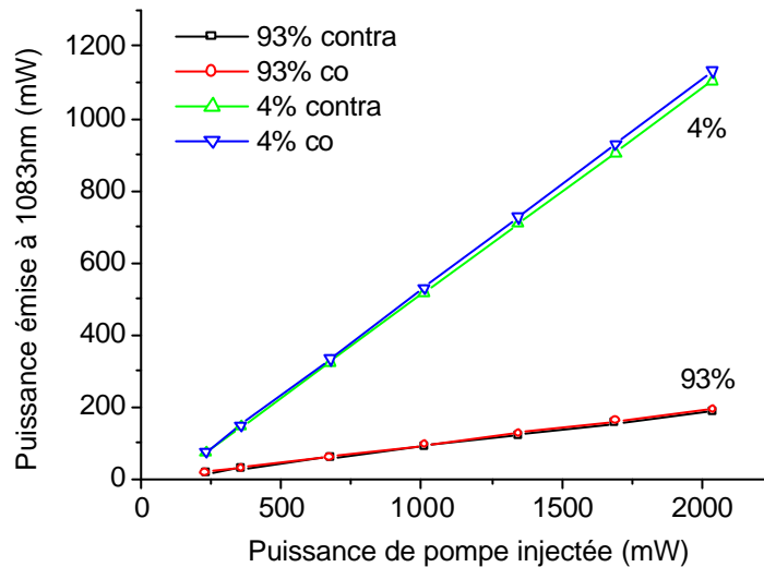
Figure III-8 Laser à 1083 nm - Puissance émise en fonction de la puissance de pompe injectée. Comparaison entre le pompage co- et contra-propagatif pour deux réflectivités de R_{min} . Pertes identiques à droite et à gauche de la fibre dopée.
