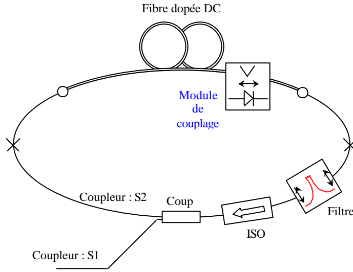
Figure II-5 Structure du laser en anneau.
