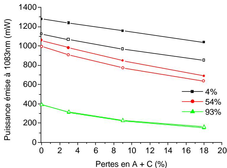
Figure III-4 : Laser à 1083 nm - Puissance émise en fonction des pertes en A + C suivant la réflectivité du miroir Rmin. Symboles pleins : Modèle numérique - Symboles vides : Modèle de M. Dignonnet
