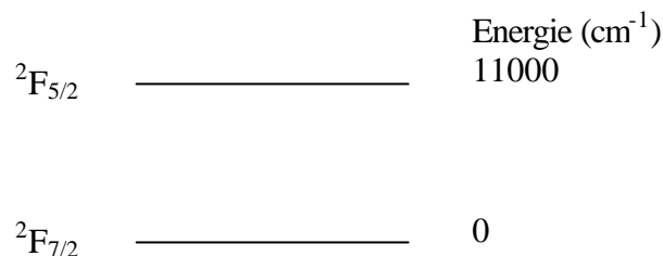
Diagramme II-1 : Niveaux d'énergie de l'ion ytterbium isolé
