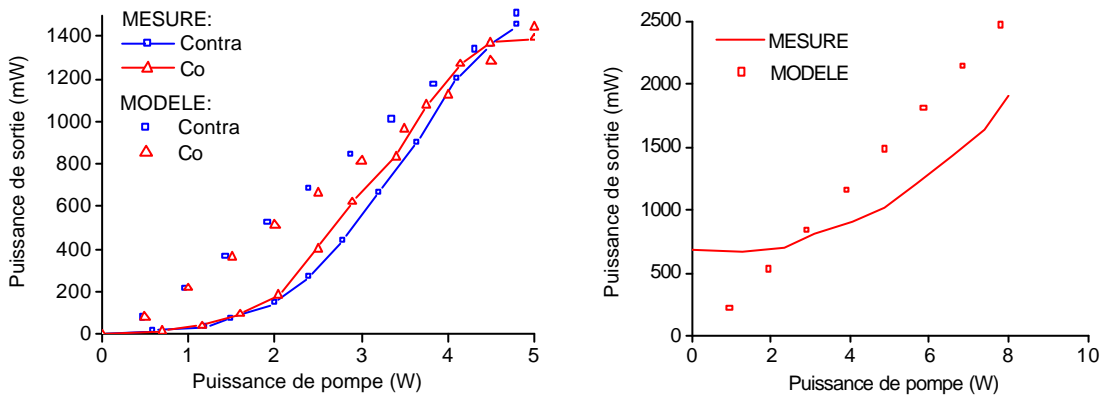
Figure III-25 à gauche : Puissance totale extraite mesurée en C dans les deux configurations en utilisant qu'un seul module de pompage.
