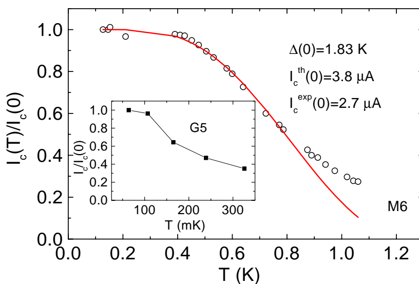
FIG. 2.8 – Courant critique de la corde M6 en fonction de la température. Les données sont compatibles avec une dépendance du type Ambegaokar-Baratoff excepté à haute température. Insert : courant critique de la corde G5 en fonction de la température.
