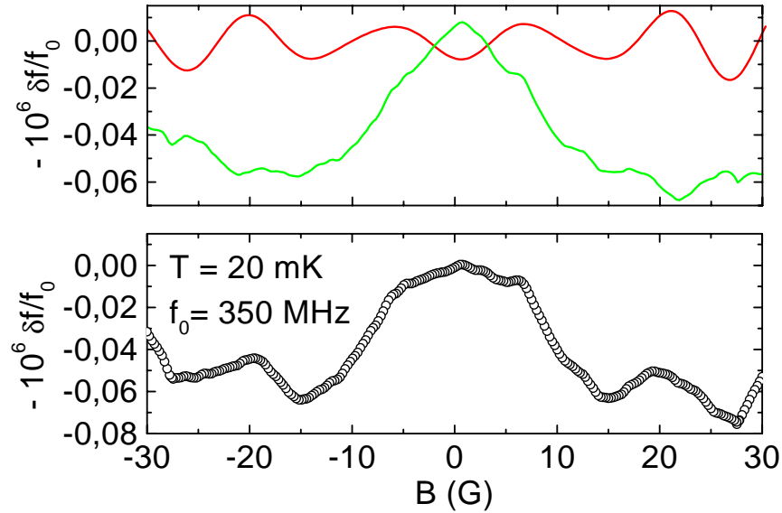
FIG. 1.2 – Courbe du bas : variation de la fréquence de résonance due aux anneaux à 20 mK et sans éclairage. Courbe du haut : le signal précédent est décomposé en une partie périodique, présentant une périodicité compatible avec un demi quantum de flux dans la surface de l’anneau, et une partie apériodique.
