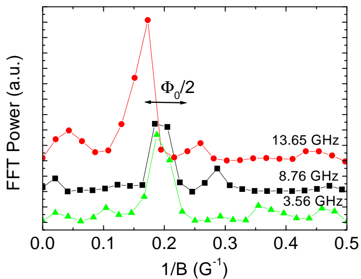
FIG. 7.10 – Transformée de Fourier de la partie impaire de l'effet PV sur la grille à 20 mK (la transformée de Fourier est faite sur une plage de champ allant de -15 à 15 G). Les courbes sont décalées pour plus de clarté.
