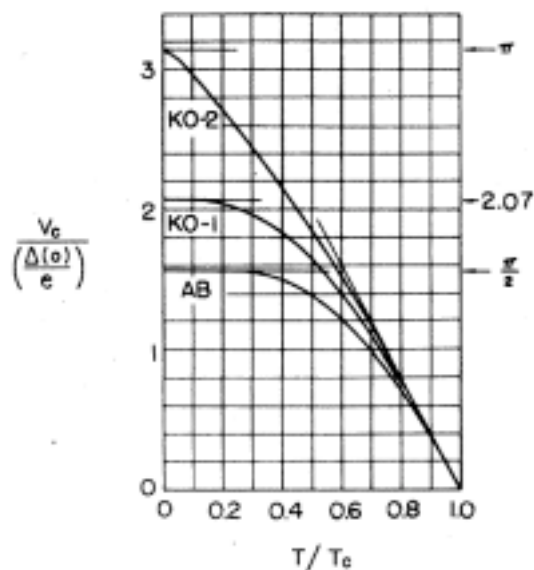
FIG. 2.14 – Dépendance en température du courant critique ( V_c = R_N I_c ) pour différents types de jonctions SNS courtes. (AB) Théorie pour une jonction tunnel (Ambegaokar et Baratoff [82]). (KO-1) Jonction diffusive (Kulik et Omelyanchuk [83]). (KO-2) Jonction balistique [84]. Cette figure est extraite de la référence [85].
