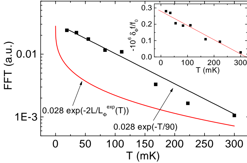
FIG. 3.4 – Dépendance en température de la composante en \Phi_0/2 du signal. L'amplitude du signal est supposée être de la forme \exp(-2L/L_\Phi(T)) . Nous avons essayé deux formes pour L_\Phi(T) : celle, notée L_\Phi^{\text{exp}}(T) , issue des expériences de localisation faible sur échantillons connectés et, d'autre part, L_\Phi(T) \propto 1/T . La dernière solution donne le meilleur accord avec les données. Insert : Dépendance en température de la variation en fréquence due aux anneaux.
