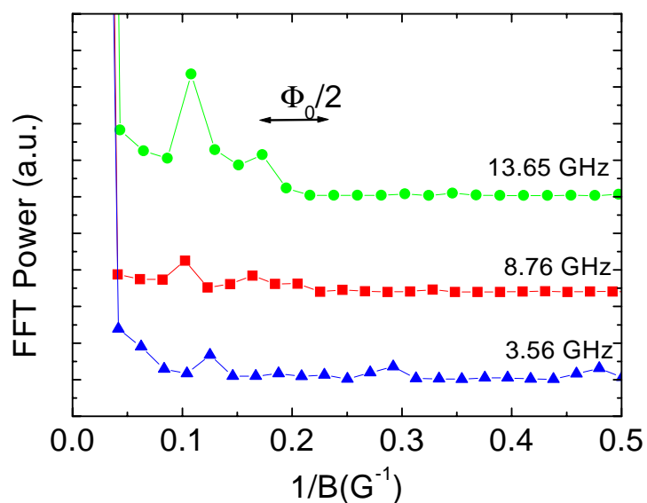
FIG. 7.11 – Transformée de Fourier de la composante paire de l'effet PV sur la grille. Les courbes sont décalées pour plus de clarté.
