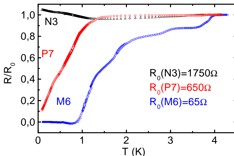
FIG. 2.1 – Dépendance des résistances des cordes N3, P7 et M6 en fonction de la température. Seule la corde M6 présente une transition vers un état de résistance nulle.
