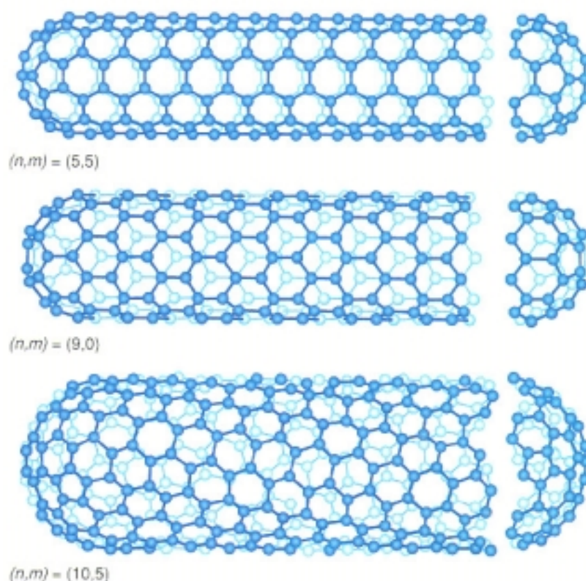
FIG. 1.2 – Différents types de nanotubes monoparois : tube armchair (5,5), tube zigzag (9,0), hélicité quelconque (10,5). On notera l'organisation transverse des atomes de carbone pour les deux premiers tubes qui est à l'origine du nom qui leur est attribué.
