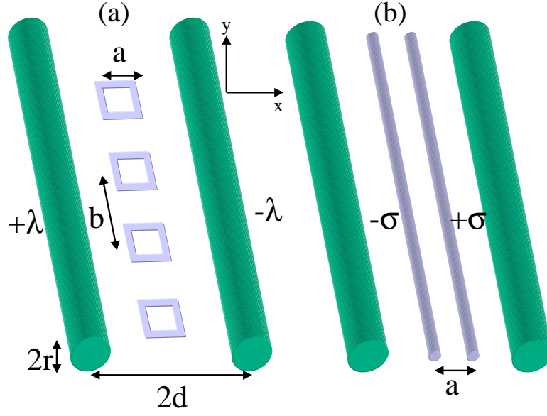
FIG. A.1 – (a) Schéma des anneaux couplés avec le résonateur. (b) Modélisation utilisée pour l'estimation du coefficient de couplage électrique. La charge linéique \sigma est déterminée par la polarisabilité des anneaux et le champ électrique généré par la capacitance à la position des anneaux.
