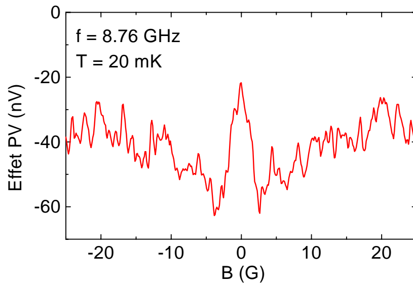
FIG. 7.8 – Effet PV sur une grille à 20 mK et 8.76 GHz.
