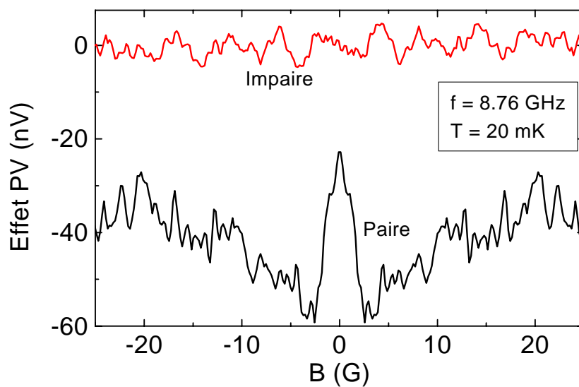
FIG. 7.9 – Décomposition de l'effet PV sur une grille à 20 mK et 8.76 GHz en sa partie paire et sa partie impaire en champ.
