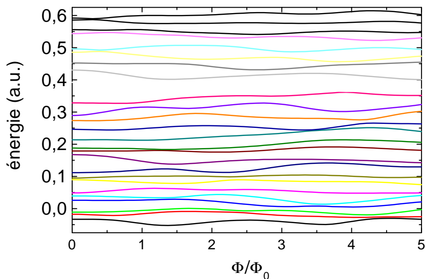
FIG. D.1 – Vue d'une partie du spectre d'un rectangle de 10 \times 20 sites avec un désordre W = 2 calculé dans le modèle d'Anderson pour différentes valeurs de flux magnétique dans la surface de l'échantillon. On notera la répulsion des niveaux induite par le désordre ainsi que les corrélations dans le spectre.
