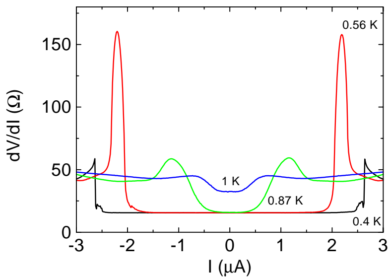
FIG. 2.5 – Résistance différentielle de M6 à différentes températures.
