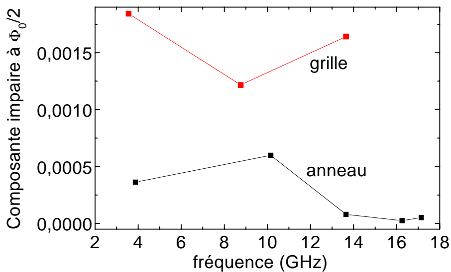
FIG. 7.13 – Rapport de la composante à \Phi_0/2 de la partie impaire et de la partie paire de l'effet PV sur la grille et sur l'anneau.
