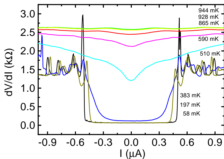
FIG. 2.7 – Résistance différentielle de G3 à différentes températures.
