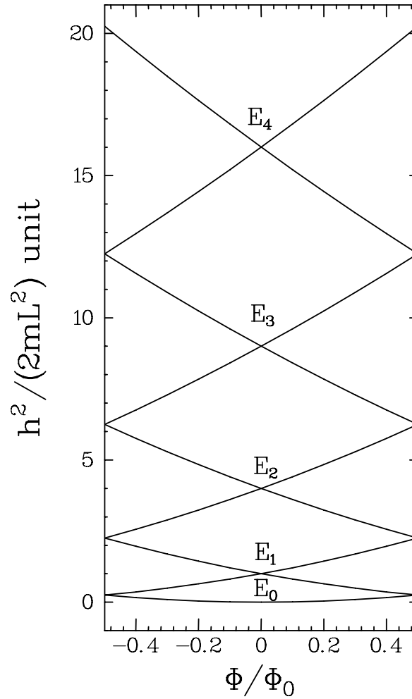
FIG. 2.8 – Niveaux d'énergie d'un anneau 1D en fonction du flux magnétique.
