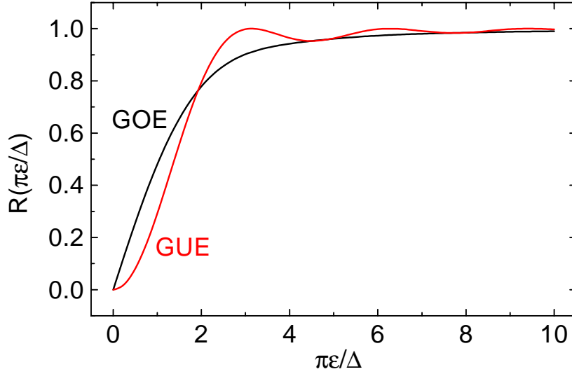
FIG. C.1 – Fonction de corrélation à deux niveaux en GOE et GUE.
