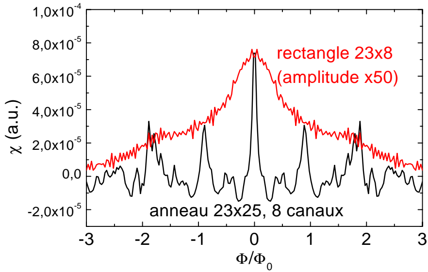
FIG. 5.2 – Susceptibilité magnétique, calculée dans le modèle d’Anderson, d’un anneau de dimension extérieure 23 \times 25 sites possédant 8 canaux, et d’un rectangle 23 \times 8 . Les deux systèmes ont un désordre de 0.7. On notera la très faible amplitude de la susceptibilité du rectangle comparée à celle de l’anneau. L’échelle de champ est fixée par le flux dans la surface maximale de l’anneau (ici 23 \times 25 ). La périodicité mesurée sur l’anneau est compatible avec un demi quantum de flux dans la surface moyenne de l’anneau.
