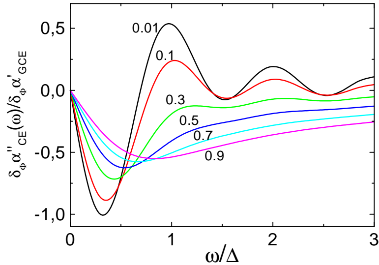
FIG. 4.3 – Valeur calculée de l'absorption électrique en CE en fonction de la fréquence à différente valeur du paramètre \gamma/\Delta
