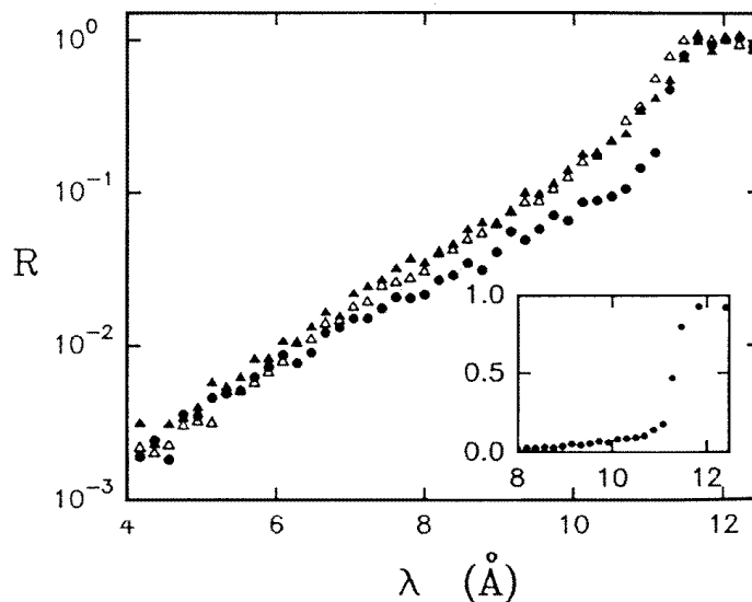
FIG. 2.3 – Réflectivité de neutrons sur la surface libre du mélange méthanol-cyclohexane deutéré. \lambda est la longueur d'onde des neutrons incidents. A l'approche du point critique (symbole ●), une "pseudo-discontinuité" par un profil de concentration en loi de puissance apparaît au bord du plateau de réflexion totale, vers 11,3 Å (d'après [46]).
